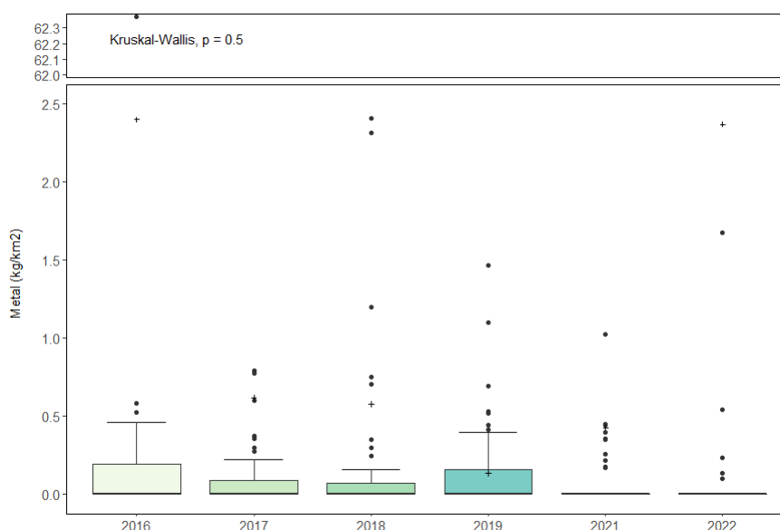
Figura 27. Abundancias de metales de fondo cuantificados durante las campañas MEDITS (kg/km 2 ). Las cajas representan la dispersión del conjunto de datos, siendo la barra superior el percentil 75, la inferior el percentil 25 y la línea central la mediana. Las barras se extienden hasta los valores extremos y los valores atípicos se representan individualmente como círculos. La media se indica con cruces (+).
