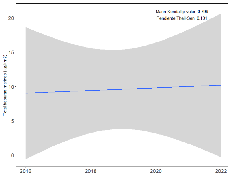
Figura 17. Análisis de la tendencia de basuras marinas (kg/km 2 ) recogidas durante las campañas y los resultados estadísticos asociados. La línea azul muestra la pendiente de las abundancias durante el periodo evaluado mediante el método no paramétrico Theil-Sen, y la banda gris su intervalo de confianza del 95 %. Un p-valor del test Mann-Kendall menor a 0,05 indica una tendencia significativa.
