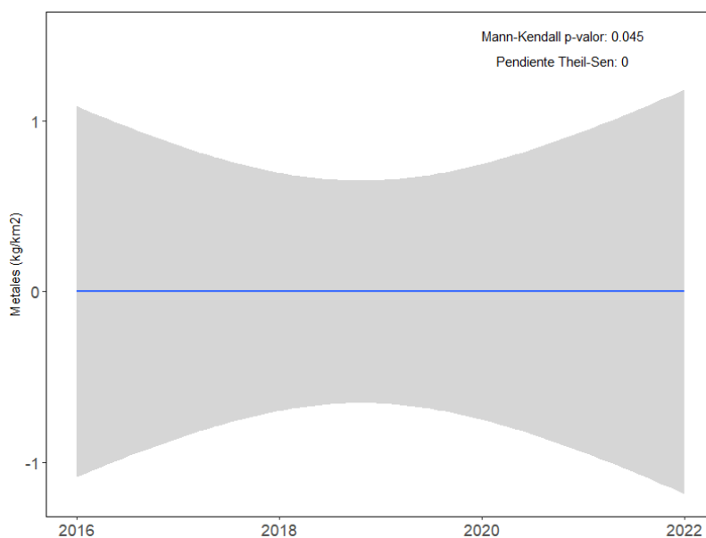
Figura 28. Análisis de la tendencia de metales (kg/km 2 ) recogidos durante las campañas y los resultados estadísticos asociados. La línea azul muestra la pendiente de las abundancias durante el periodo evaluado mediante el método no paramétrico Theil-Sen, y la banda gris su intervalo de confianza del 95 %. Un p -valor del test Mann-Kendall menor a 0,05 indica una tendencia significativa.
