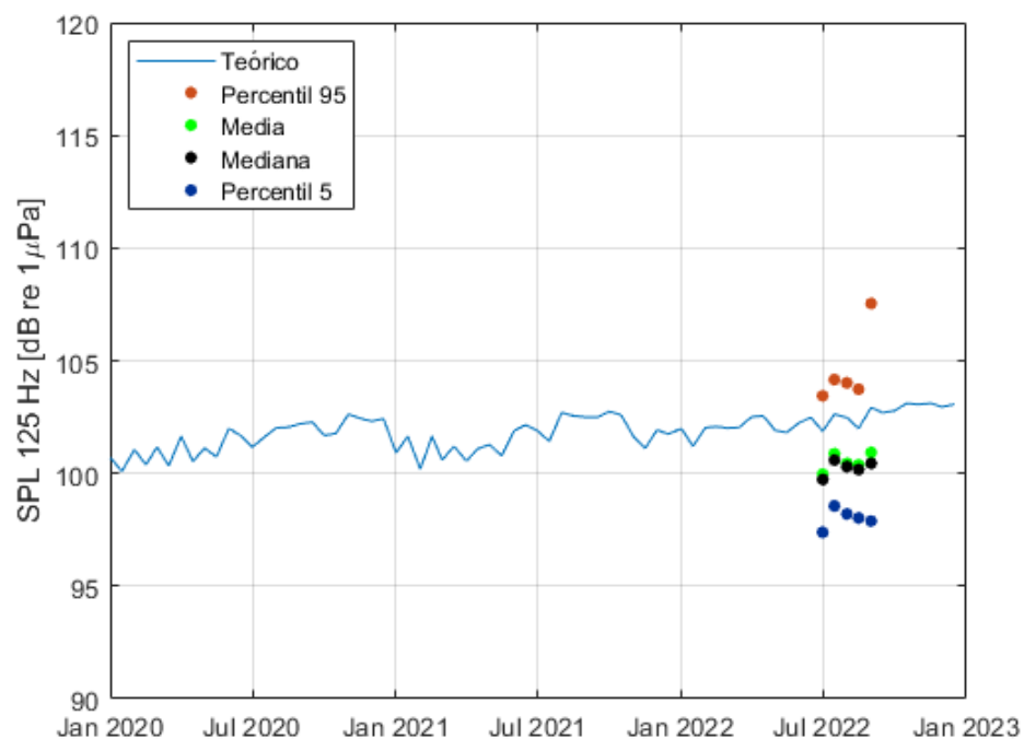
Figura 22. Curva teórica obtenida en la banda de \frac{1}{3} de octava de 125 Hz en la localización del fondeo situado en los escarpes de Mazarrón y puntos correspondientes a media aritmética (verde) y a los percentiles 5, 50 y 95 (azul, negro y naranja respectivamente) quincenales de las medidas experimentales.
