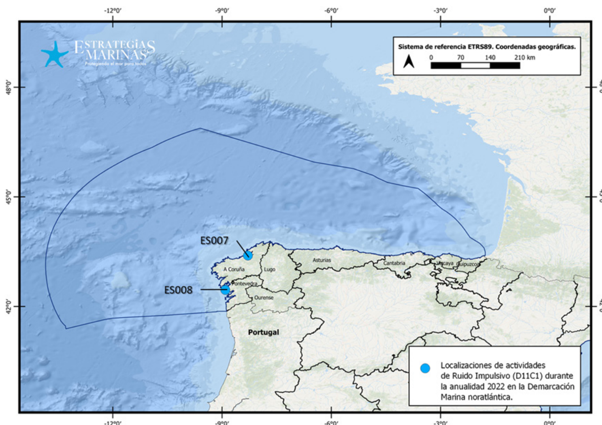
Figura 3. Localización de actividades generadoras de sonido impulsivo llevadas a cabo durante la anualidad 2022 en la demarcación marina noratlántica.
