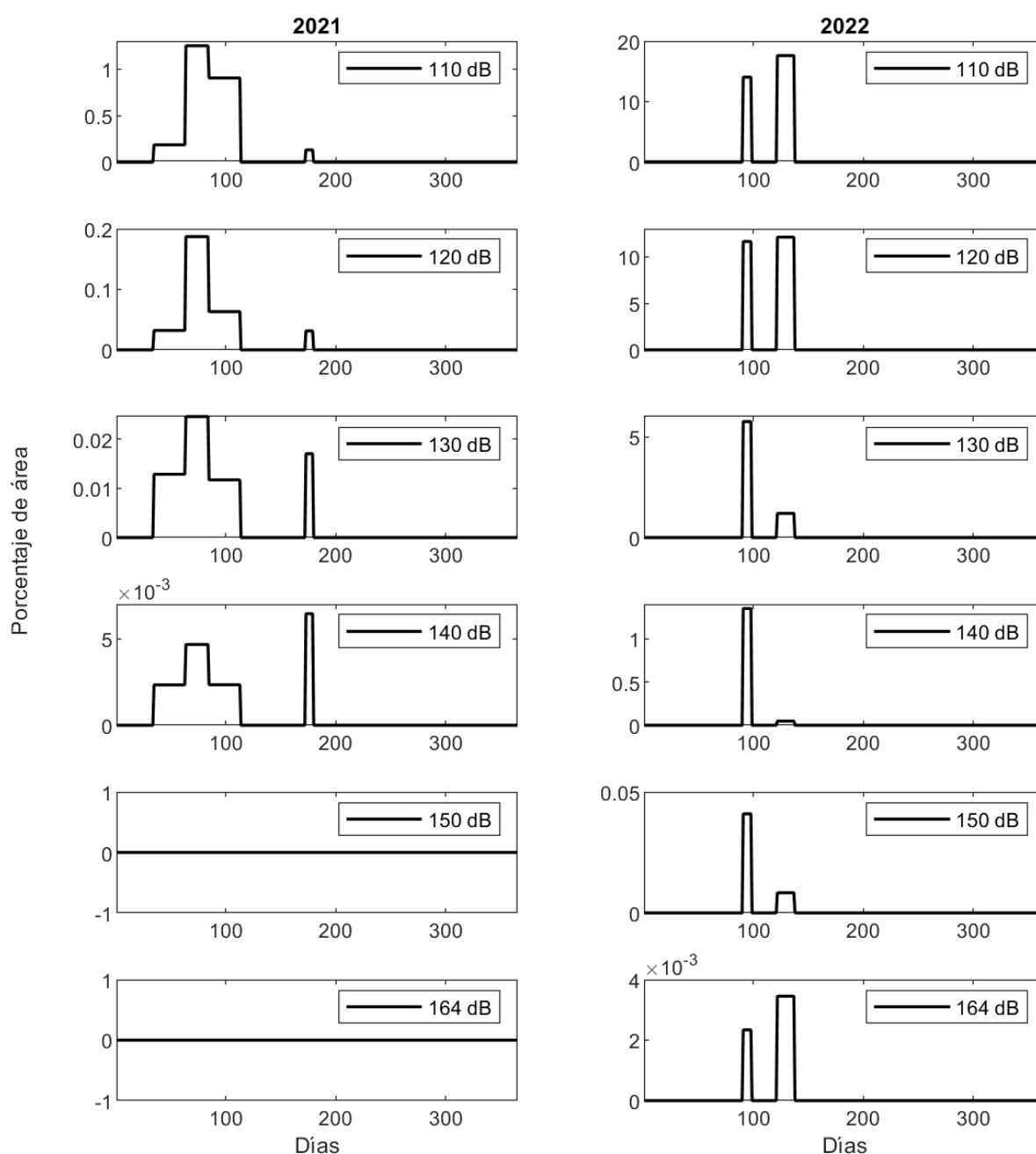
Figura 17. Porcentaje de área de la demarcación marina noratlántica que presenta un nivel de exposición sonora superior a diversos niveles considerados (indicados en la leyenda) para cada día de las dos anualidades evaluadas.
