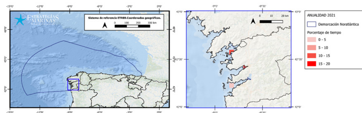
Figura 4. Porcentaje de días con actividad generadora de sonido impulsivo en cada celda ( C\text{-Square} de 0,05^{\circ} \times 0,05^{\circ} ) en la demarcación noratlántica en 2021.
