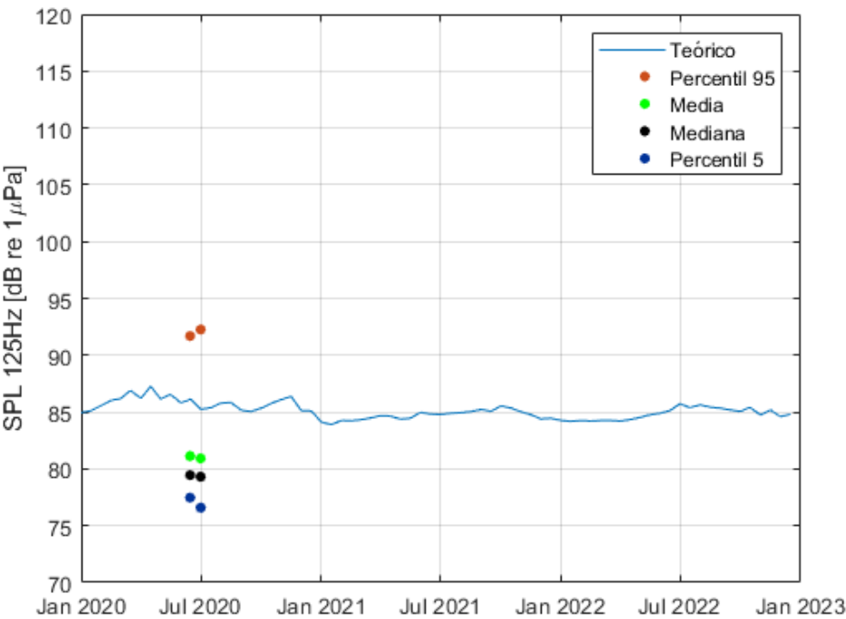
Figura 28. Curva teórica obtenida en la banda de \frac{1}{3} de octava de 125 Hz en la localización del fondeo situado en el golfo de Vizcaya y puntos correspondientes a media aritmética (verde) y a los percentiles 5, 50 y 95 (azul, negro y naranja respectivamente) quincenales de las medidas experimentales.
