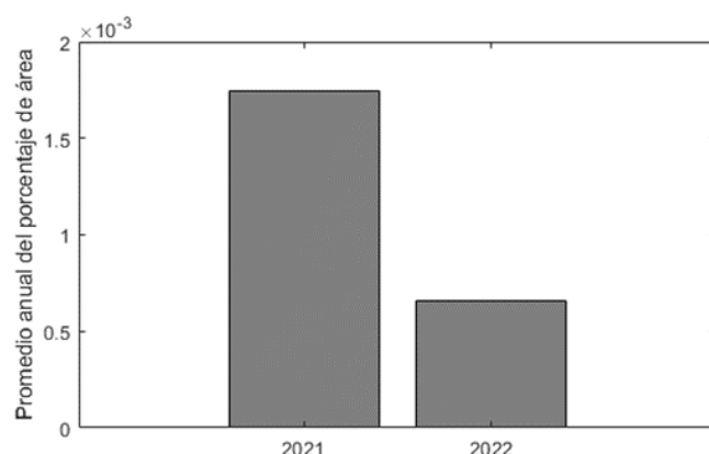
Figura 11. Promedio anual en base mensual del porcentaje de área con presencia de actividades generadoras de sonido impulsivo en la demarcación marina noratlántica.
