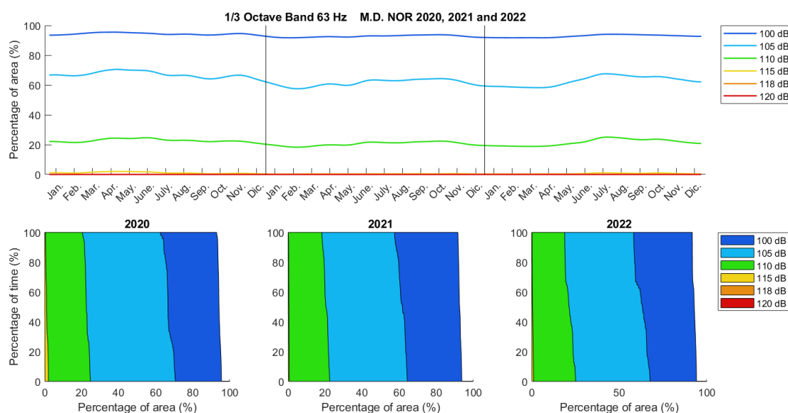
Figura 33. (superior) Evolución durante el periodo de evaluación del porcentaje de área que se encuentra por encima de los distintos valores de nivel considerados como umbral y que a futuro deberán determinar la potencial afección sobre especies indicadoras (LOBE). (Inferior) Curvas de porcentaje de tiempo, relacionadas con el porcentaje de área por encima de los distintos umbrales de nivel (en base anual)
