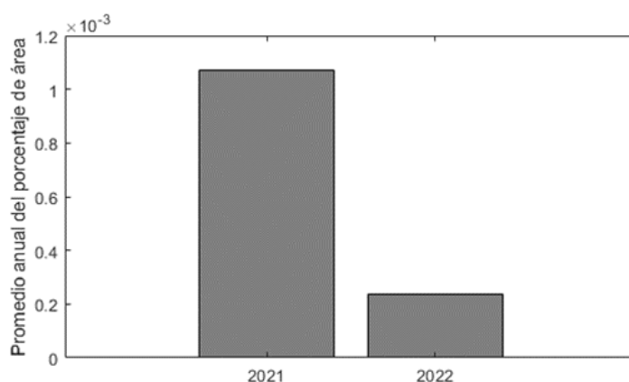
Figura 9. Promedio anual en base diaria del porcentaje de área con presencia de actividades generadoras de sonido impulsivo en la demarcación marina noratlántica.
