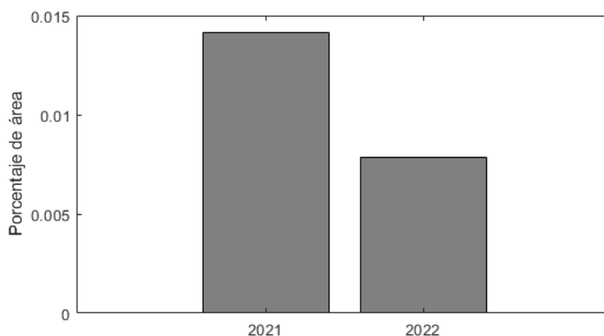
Figura 7. Porcentaje de área con fuentes de sonido impulsivas en la demarcación noratlántica en 2021 y 2022.
