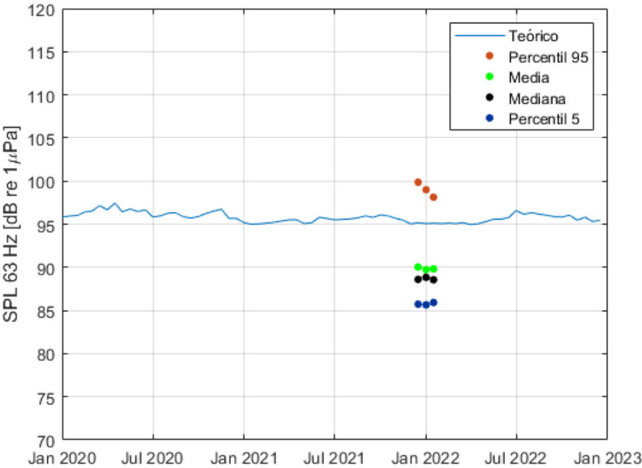
Figura 29. Curva teórica obtenida en la banda de \frac{1}{3} de octava de 63 Hz en la localización del fondeo situado al oeste del monte submarino del Cachucho (Cachucho A) y puntos correspondientes a media aritmética (verde) y a los percentiles 5, 50 y 95 (azul, negro y naranja respectivamente) quincenales de las medidas experimentales.
