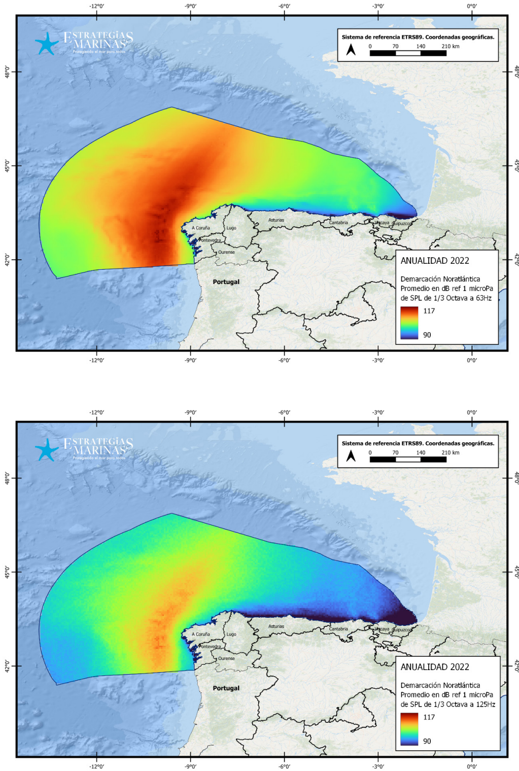
Figura 21. Valor medio anual en base temporal horaria del nivel de sonido calculado en la banda de frecuencia de tercio de octava de 63 y 125 Hz correspondiente a la anualidad 2022 [dB ref 1 \mu Pa].
