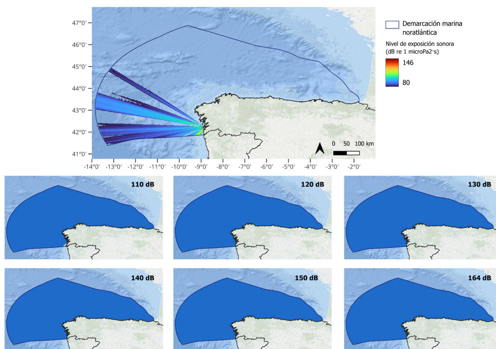
Figura 13. Mapa de nivel de exposición sonora generado por el hincado de pilotes de la actividad registrada como ES002 en la demarcación marina noratlántica en la anualidad 2021. En miniatura se representa el área que presenta niveles de exposición sonora superiores (amarillo) e inferiores (azul) para los diferentes valores de umbral de SEL considerados (indicados en la leyenda de cada mapa).
