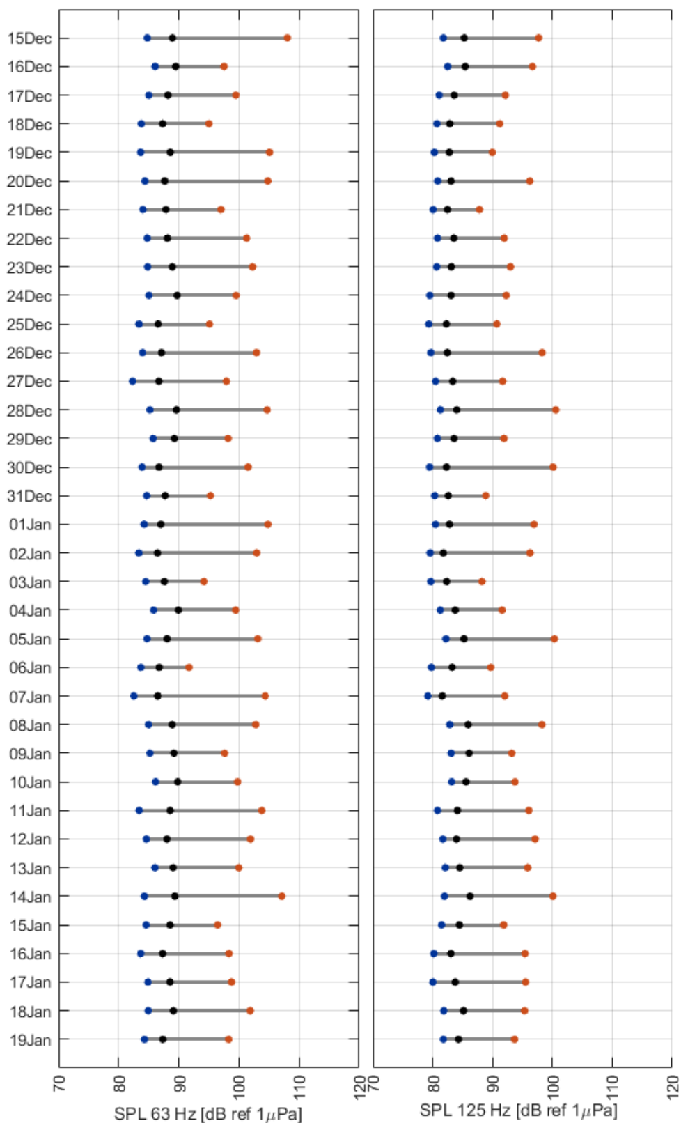
Figura 25. Gráfica correspondiente a las medidas experimentales en el punto de monitorización situado al oeste del monte submarino del Cachucho. A partir de los datos de nivel de presión sonora [db ref 1 \mu Pa] obtenidos cada 2 segundos se han calculado los percentiles 5 (en puntos azules), 50 (en puntos negros) y 95 (puntos naranjas) diarios en las bandas de frecuencias de tercio de octava de 63 y 125 Hz.
