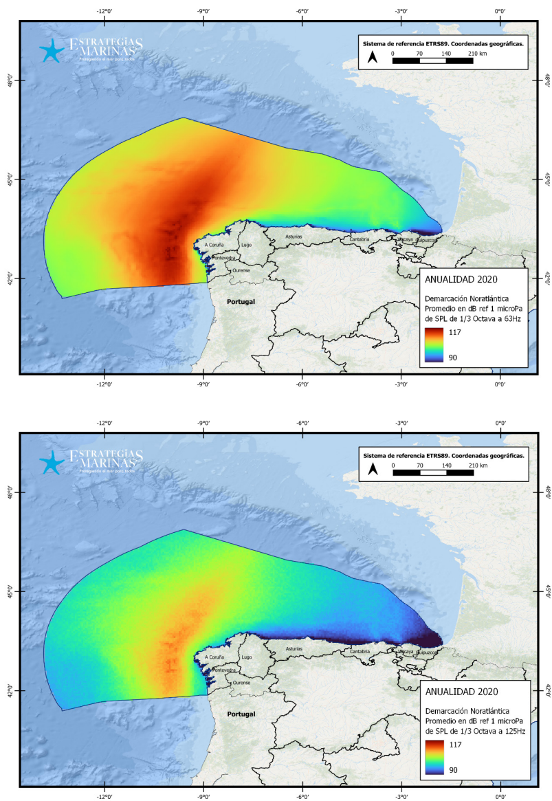
Figura 19. Valor medio anual en base temporal horaria del nivel de sonido calculado en la banda de frecuencia de tercio de octava de 63 y 125 Hz correspondiente a la anualidad 2020 [dB ref 1 µPa].
