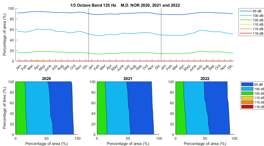
Figura 34. (superior) Evolución durante el periodo de evaluación del porcentaje de área que se encuentra por encima de los distintos valores de nivel considerados como umbral y que a futuro deberán determinar la potencial afección sobre especies indicadoras (LOBE). (Inferior) Curvas de porcentaje de tiempo, relacionadas con el porcentaje de área por encima de los distintos umbrales de nivel (en base anual).
