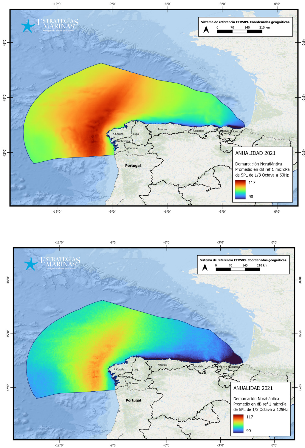
Figura 20. Valor medio anual en base temporal horaria del nivel de sonido calculado en la banda de frecuencia de tercio de octava de 63 y 125 Hz correspondiente a la anualidad 2021 [dB ref 1 \mu Pa].
