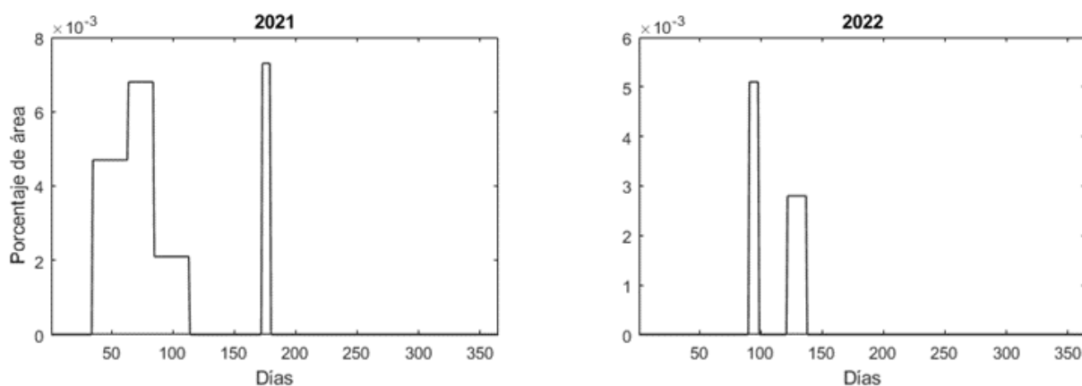
Figura 8. Porcentaje de área con presencia de actividades generadoras de sonido impulsivo de cada día de las anualidades 2021 y 2022 en la demarcación noratlántica en 2022.
