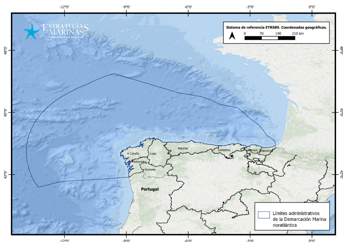
Figura 1. Detalle de la demarcación marina noratlántica en la que se ha realizado la determinación del ruido submarino siguiendo los criterios D11C1 y D11C2.
