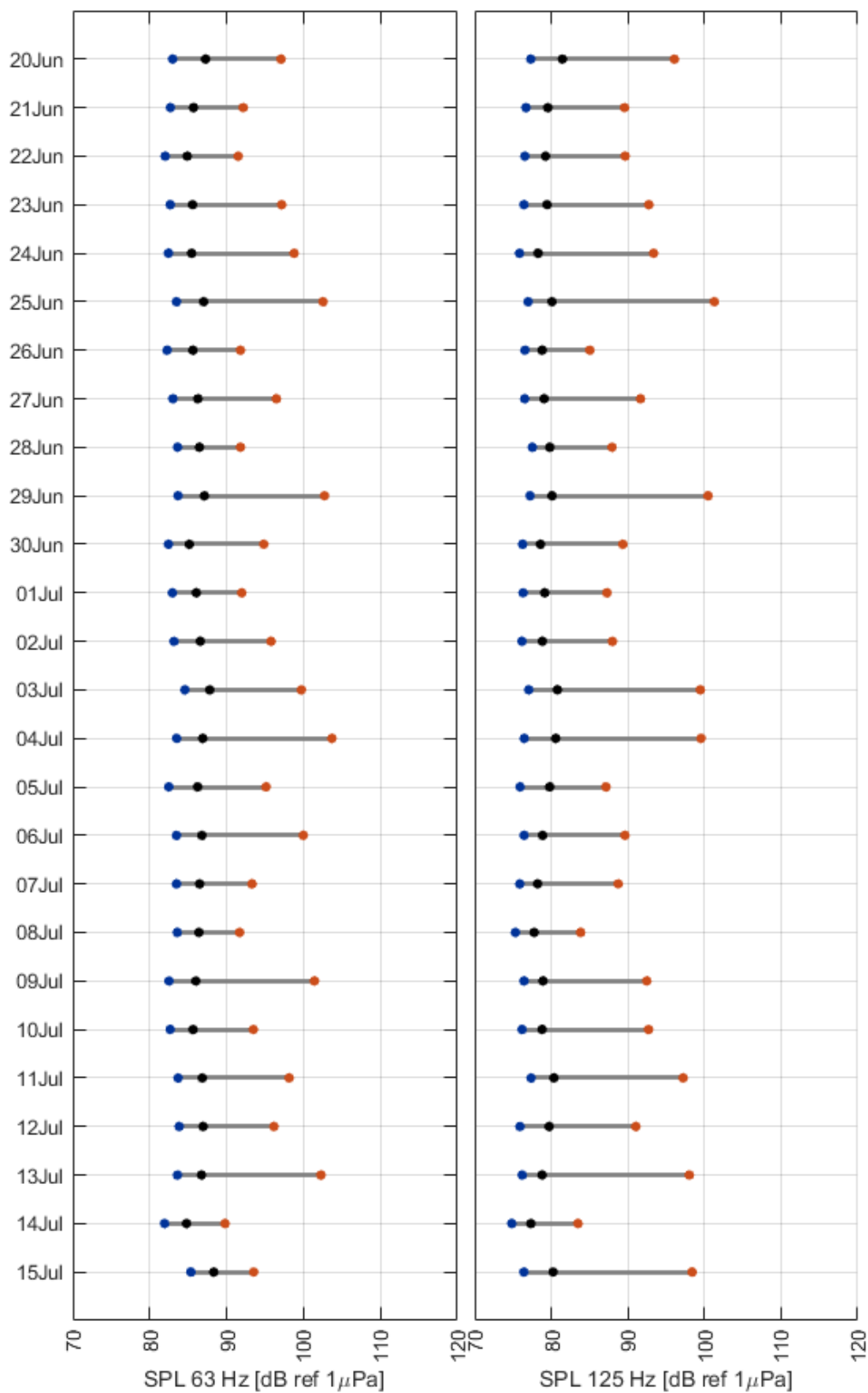
Figura 24. Gráfica correspondiente a las medidas experimentales en el punto de monitorización situado en el golfo de Vizcaya. A partir de los datos de nivel de presión sonora [db ref 1 \mu Pa] obtenidos cada 2 segundos se han calculado los percentiles 5 (en puntos azules), 50 (en puntos negros) y 95 (puntos naranjas) diarios en las bandas de frecuencias de tercio de octava de 63 y 125 Hz.
