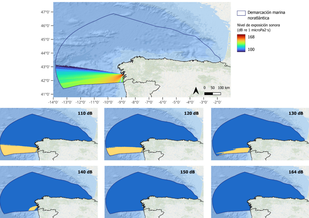
Figura 16. Mapa de nivel de exposición sonora generado por la explosión de la actividad registrada como ES008 en la demarcación marina noratlántica en la anualidad 2022. En miniatura se representa el área que presenta niveles de exposición sonora superiores (amarillo) e inferiores (azul) para los diferentes valores de umbral de SEL considerados (indicados en la leyenda de cada mapa).
