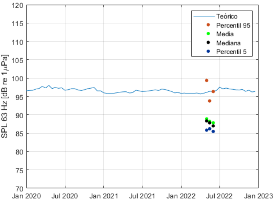
Figura 31. Curva teórica obtenida en la banda de \frac{1}{3} de octava de 63 Hz en la localización del fondeo situado al este del monte submarino del Cachucho (Cachucho B) y puntos correspondientes a media aritmética (verde) y a los percentiles 5, 50 y 95 (azul, negro y naranja respectivamente) quincenales de las medidas experimentales.
