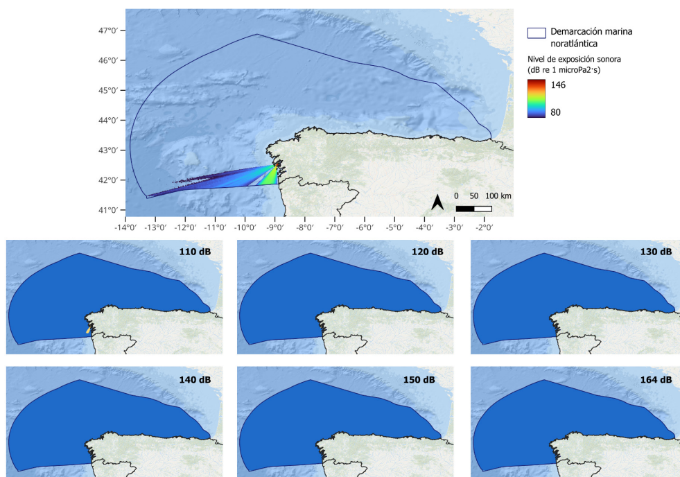
Figura 14. Mapa de nivel de exposición sonora generado por el hincado de pilotes de la actividad registrada como ES003 en la demarcación marina noratlántica en la anualidad 2021. En miniatura se representa el área que presenta niveles de exposición sonora superiores (amarillo) e inferiores (azul) para los diferentes valores de umbral de SEL considerados (indicados en la leyenda de cada mapa).
