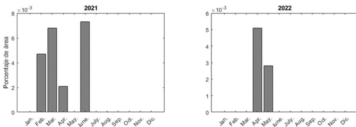
Figura 10. Porcentaje de área con presencia de actividades generadoras de sonido impulsivo de cada mes de las anualidades 2021 y 2022 en la demarcación noratlántica.
