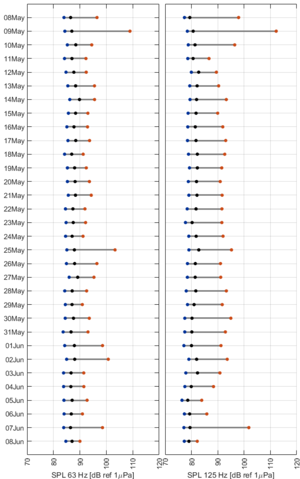
Figura 26. Gráfica correspondiente a las medidas experimentales en el punto de monitorización situado al este del monte submarino del Cachucho. A partir de los datos de nivel de presión sonora [dB ref 1 \mu Pa] obtenidos cada 2 segundos se han calculado los percentiles 5 (en puntos azules), 50 (en puntos negros) y 95 (puntos naranjas) diarios en las bandas de frecuencias de tercio de octava de 63 y 125 Hz.
