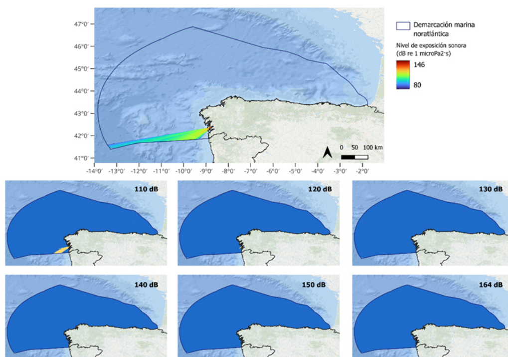
Figura 12. Mapa de nivel de exposición sonora generado por el hincado de pilotes de la actividad registrada como ESO01 en la demarcación marina noratlántica en la anualidad 2021. En miniatura se representa el área que presenta niveles de exposición sonora superiores (amarillo) e inferiores (azul) para los diferentes valores de umbral de SEL considerados (indicados en cada uno de los mapas).
