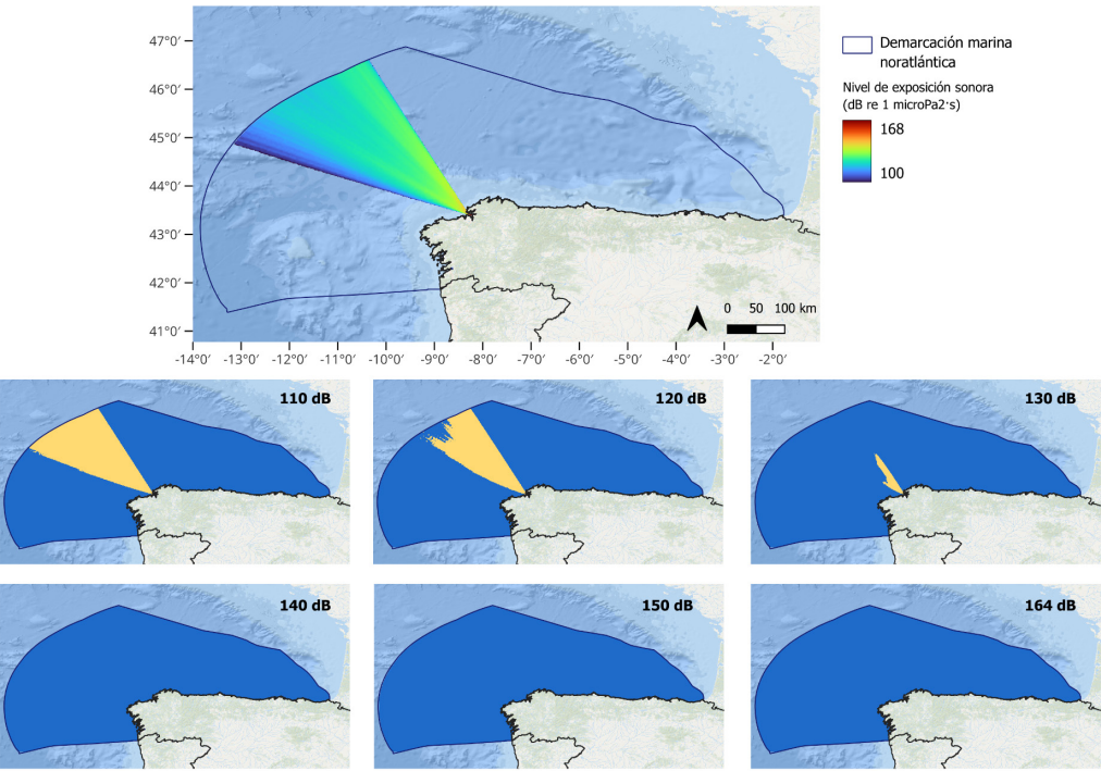
Figura 15. Mapa de nivel de exposición sonora generado por la explosión de la actividad registrada como ES007 en la demarcación marina noratlántica en la anualidad 2022. En miniatura se representa el área que presenta niveles de exposición sonora superiores (amarillo) e inferiores (azul) para los diferentes valores de umbral de SEL considerados (indicados en la leyenda de cada mapa).
