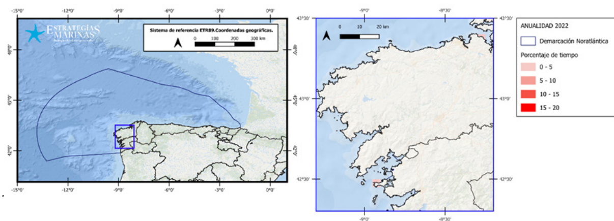
Figura 5. Porcentaje de días con actividad generadora de sonido impulsivo en cada celda ( C\text{-Square} de 0,05^{\circ} \times 0,05^{\circ} ) en la demarcación noratlántica en 2022
