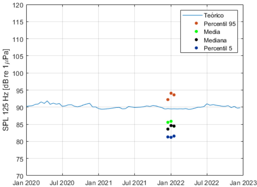
Figura 30. Curva teórica obtenida en la banda de \frac{1}{3} de octava de 125 Hz en la localización del fondeo situado al oeste del monte submarino del Cachucho (Cachucho A) y puntos correspondientes a media aritmética (verde) y a los percentiles 5, 50 y 95 (azul, negro y naranja respectivamente) quincenales de las medidas experimentales.
