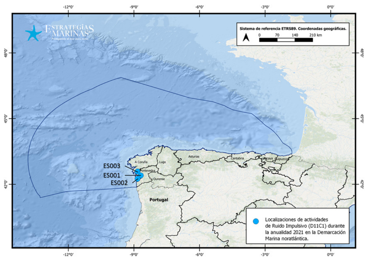
Figura 2. Localización de actividades generadoras de sonido impulsivo llevadas a cabo durante la anualidad 2021 en la demarcación marina noratlántica.
