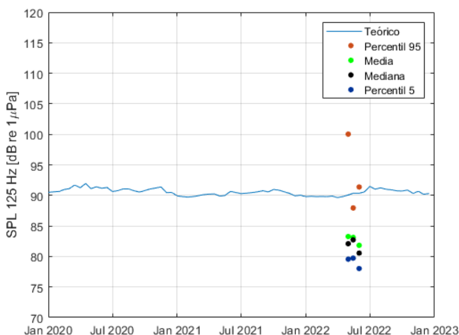
Figura 32. Curva teórica obtenida en la banda de \frac{1}{3} de octava de 63 Hz en la localización del fondeo situado al este del monte submarino del Cachucho (Cachucho B) y puntos correspondientes a media aritmética (verde) y a los percentiles 5, 50 y 95 (azul, negro y naranja respectivamente) quincenales de las medidas experimentales.
