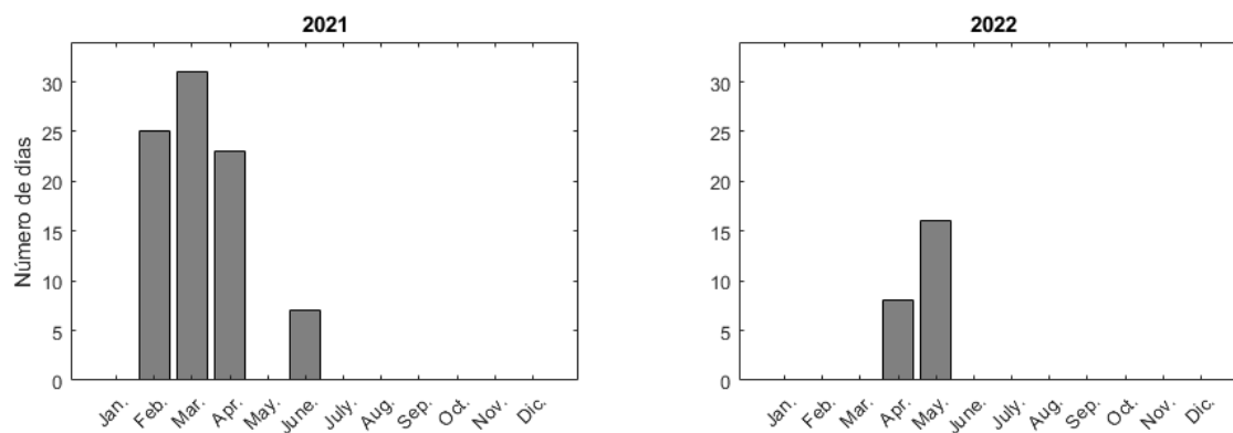
Figura 6. Número de días por mes con fuentes de sonido impulsivas en la demarcación noratlántica en 2021 y 2022.
