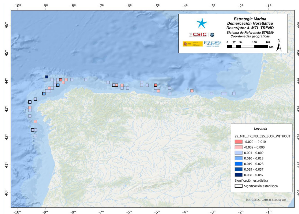
Figura 12. Talud: valores promedio del indicador por celda (arriba) y tendencia (abajo), correspondiente al escenario para mesopredadores y depredadores apicales (MTL3.25) sin pelágicos. Las celdas enmarcadas en negra representan tendencias significativas de los modelos.
