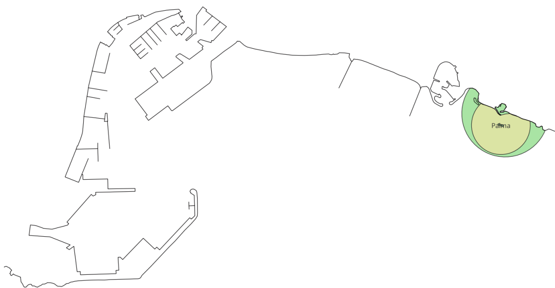
Figura 7. Actuación (verde oscuro) y zona potencialmente afectada (buffer, amarillo) por la modificación portuaria realizada en la costa de Palma. El buffer calculado para esta estructura solapa con el obtenido para la actuación que se muestra en la Figura 2.
