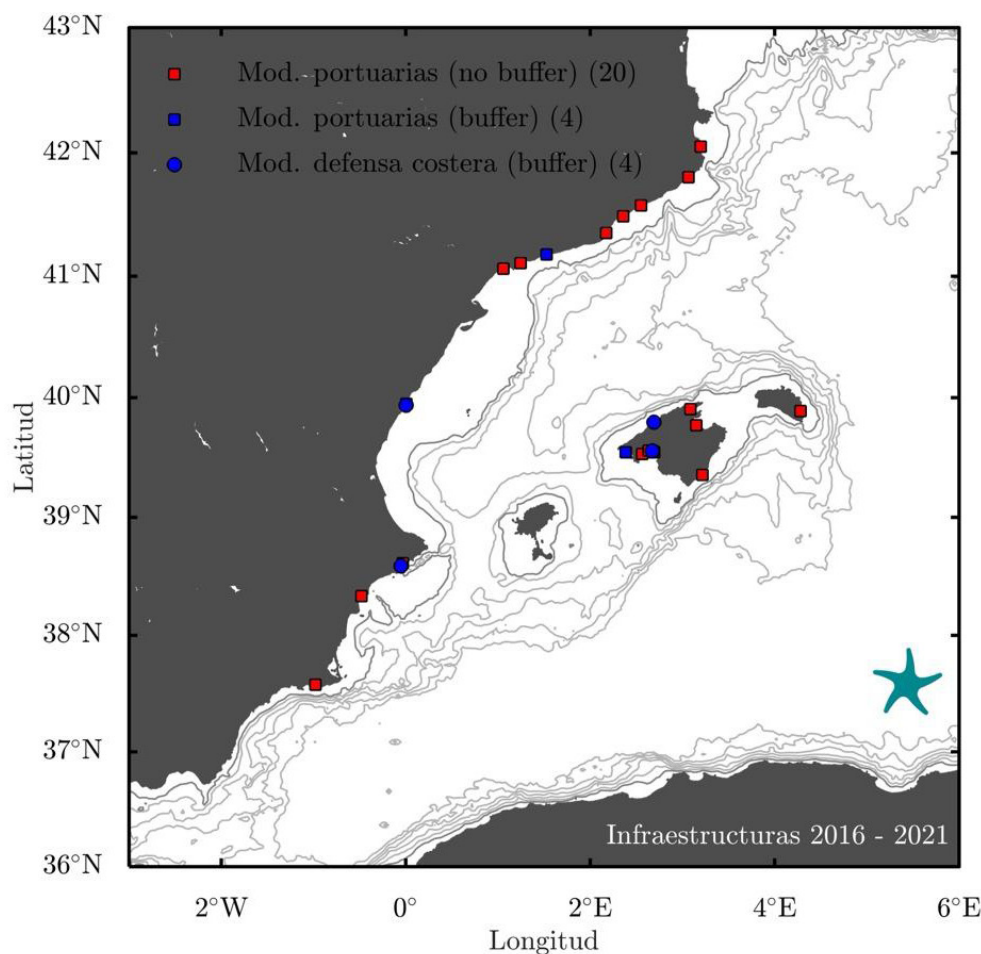
Figura 1. Obras civiles identificadas en la demarcación que pueden generar alteración hidrográfica en el periodo de estudio 2016-2021.
