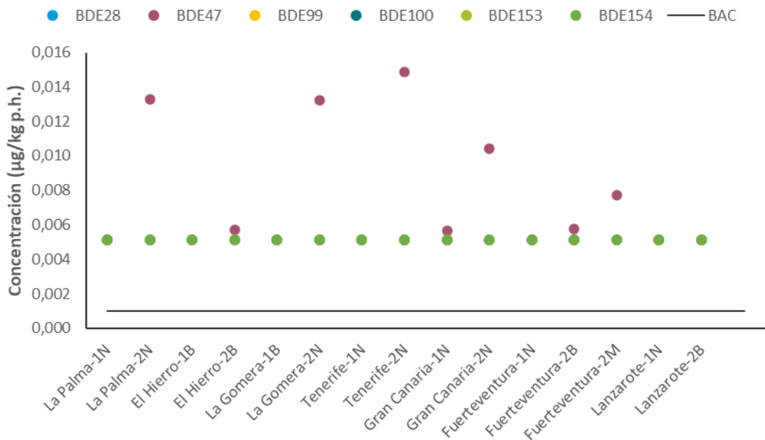
Figura 8. Concentración de los BDEs 28, 47, 99, 100, 153 y 154 en lapa/mejillón de la demarcación canaria año en 2021 (último año muestreado y analizado) y el valor BAC (0,00091 µg/kg p.h.) para todos ellos. N= negra; B= blanca y M= mejillón.
