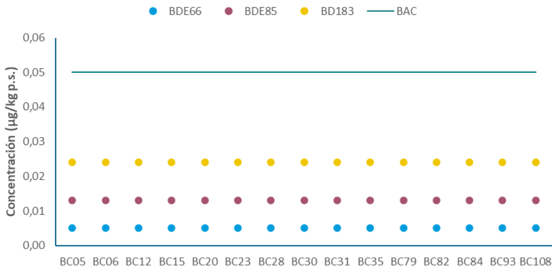
Figura 28. Concentración de los BDEs 66, 85 y 183 en los sedimentos de la plataforma continental recogidos en la demarcación del último año muestreado y analizado y el valor BAC (0,05 µg/kg p.s.) para todos ellos.
