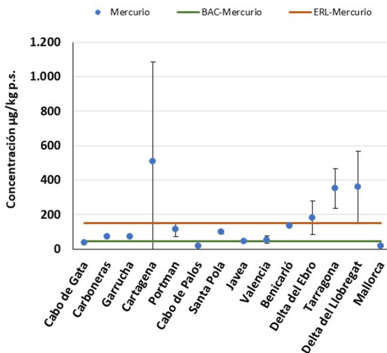
Figura 17. Concentración (valor medio \pm desviación estándar) de mercurio uPBT en sedimento marino del área PC de la DMLEBA ( \mu\text{g/kg} p.s.) muestreados los años 2013, 2014, 2015 y 2016, y el valor BAC y ERL.
