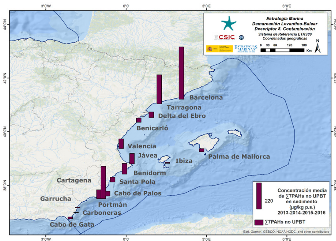
Figura 35. Distribuci n espacial del valor medio de la concentraci n del sumatorio de 7 PAHs no uPBT ( g/kg p.s.) en sedimento marino del  rea PC de la DMLEBA muestreados los  a os 2013, 2014, 2015 y 2016. \Sigma 7PAHs: fenantreno + antraceno + fluoranteno + pireno + benzo(a)antraceno + criseno + dibenzo(a,h)antraceno.
