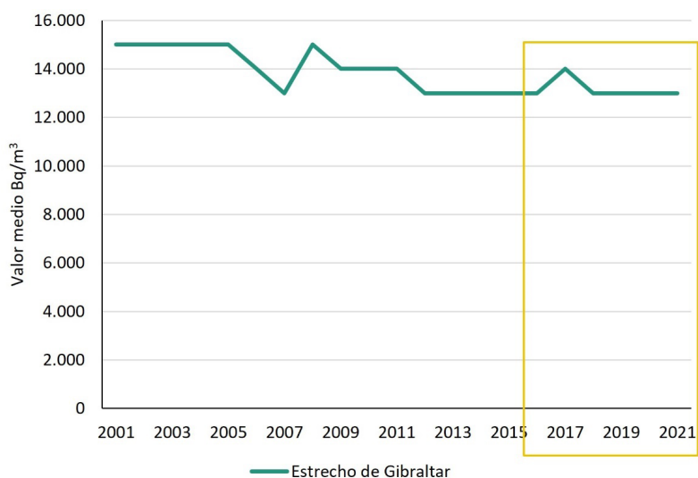
Figura 51. Concentración del índice de actividad beta total ( Bq/m^3 ) en las estaciones de la demarcación. (Fuente: Figura elaborada por el CEDEX con datos publicados por el Consejo de Seguridad Nuclear)
