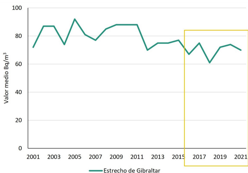
Figura 50. Concentración del índice de actividad alfa total ( Bq/m^3 ) en las estaciones de la demarcación. (Fuente: Figura elaborada por el CEDEX con datos publicados por el Consejo de Seguridad Nuclear)
