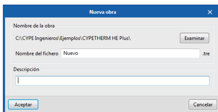
Fig. 66. Nuevo fichero
