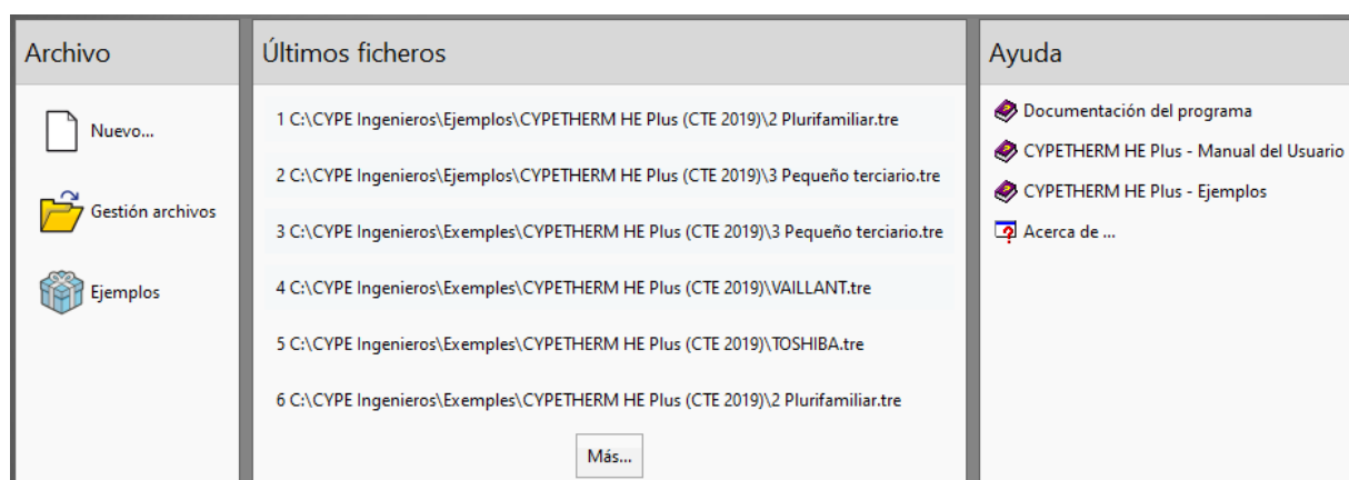
Fig. 1. Pantalla inicial
