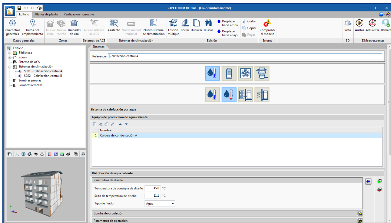
Fig. 41. Edición de un sistema de producción centralizado
