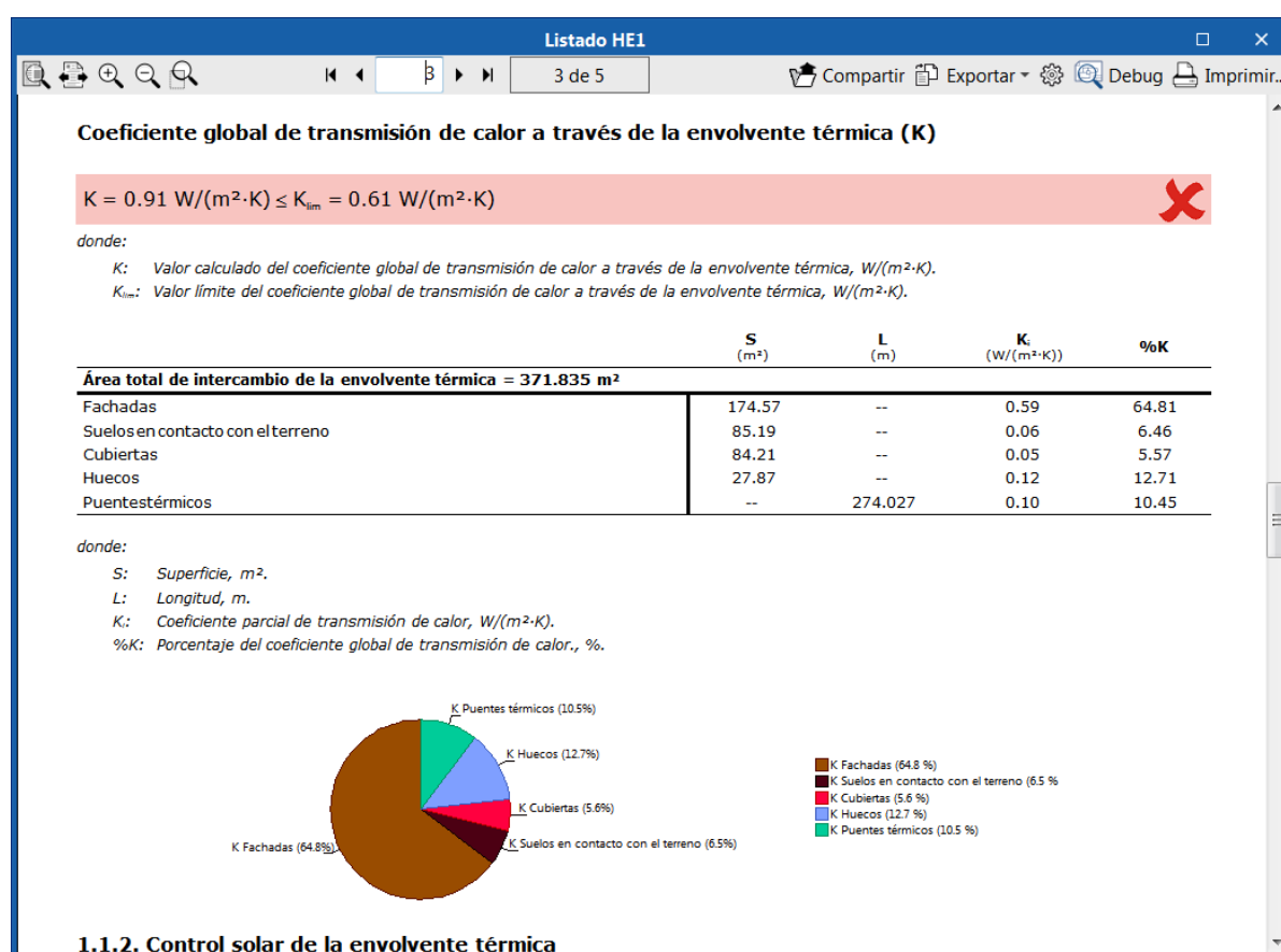
Fig. 65. Listado HE1
