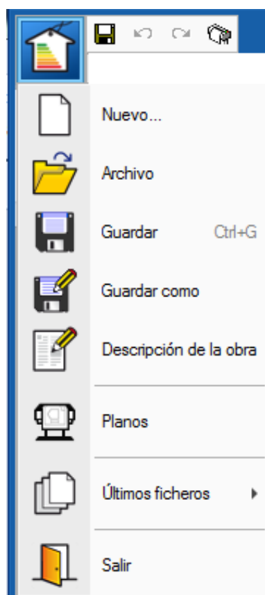
Fig. 3. Menú principal
