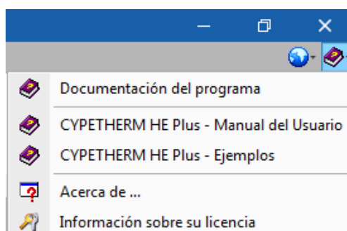
Fig. 6. Menú ayuda
