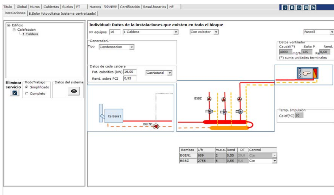
Imagen 2.40 Instalación calefacción solo detalle datos defecto
