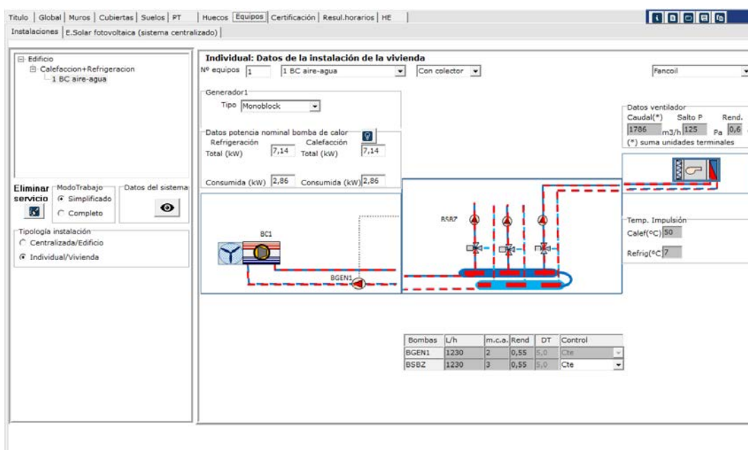
Imagen 2.48 Instalación calefacción+refrigeración. Bomba de calor aire-agua
