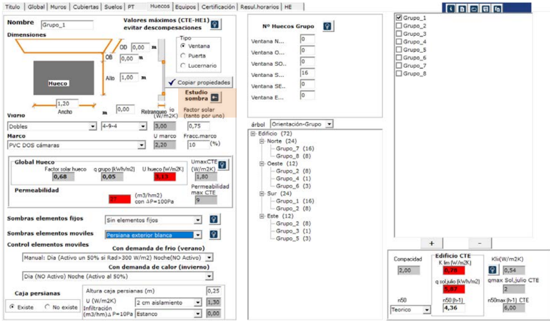
Imagen 2.21 Botón para Estudio de Sombra
