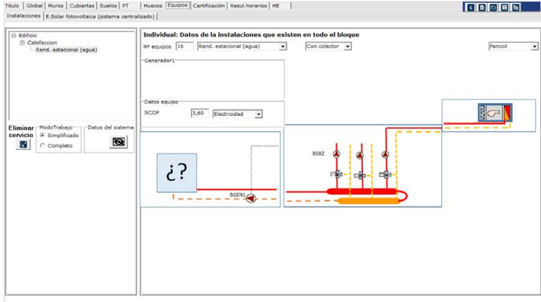
Imagen 2.41 Instalación calefacción sólo. Rendimiento estacional (agua)
