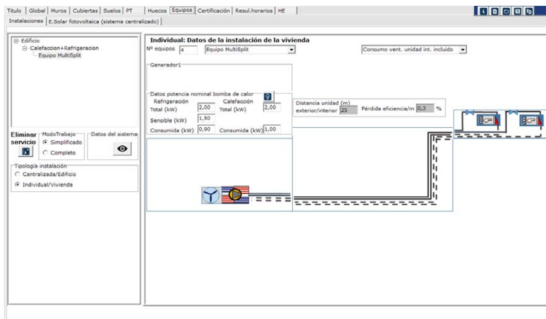
Imagen 2.46 Instalación calefacción+refrigeración. Equipo multisplit
