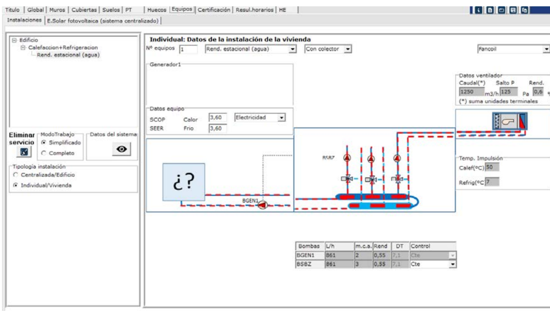
Imagen 2.49 Instalación calefacción+refrigeración. Rendimiento estacional (agua)
