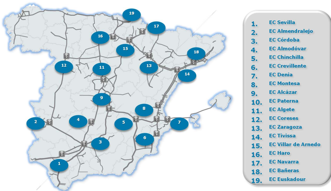
Figura 16: Estaciones de compresión del Sistema Gasista español
