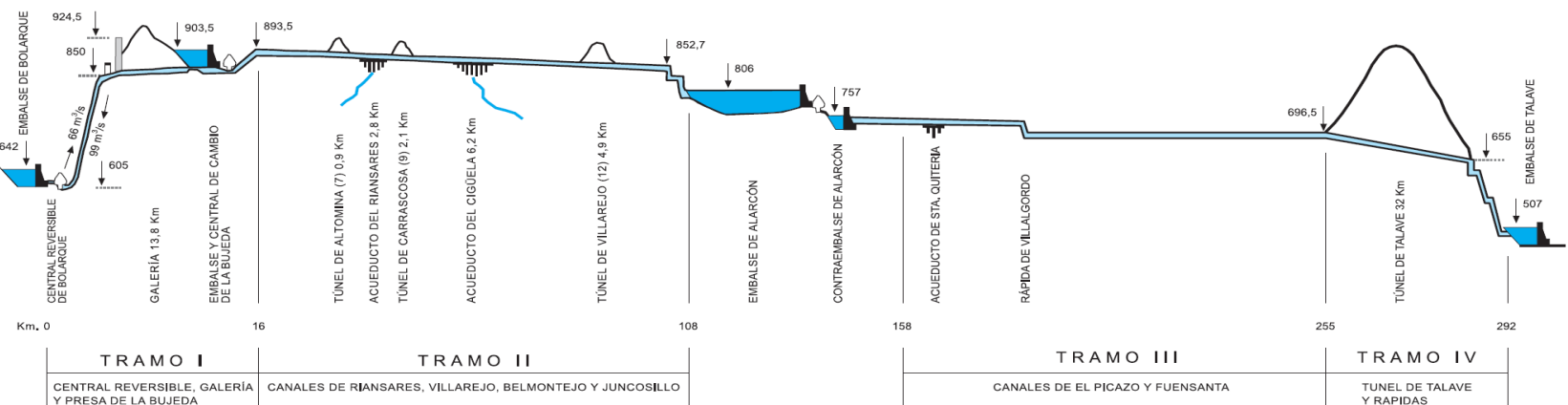
Figura 1. Perfil del trazado del Acueducto Tajo-Segura
