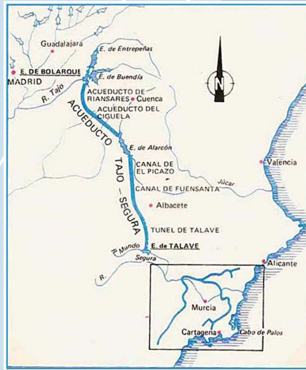
Figura 1. Perfil del trazado del Acueducto Tajo-Segura
