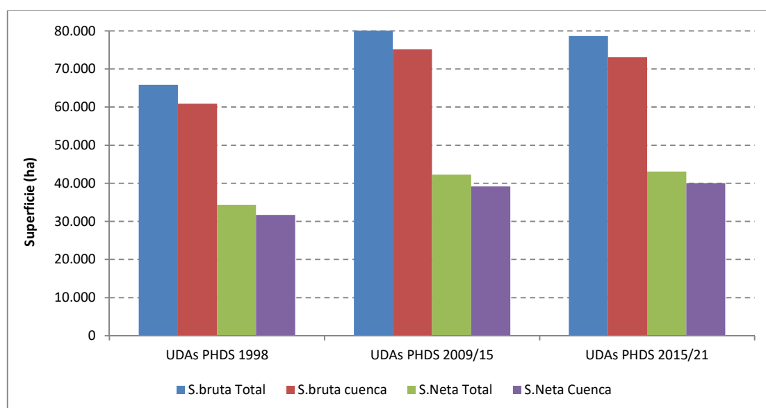
Figura 23: Evolución de superficies en UDAs en la cuenca vertiente del Mar Menor (Fuente: Elaboración propia basada en datos CHS).
