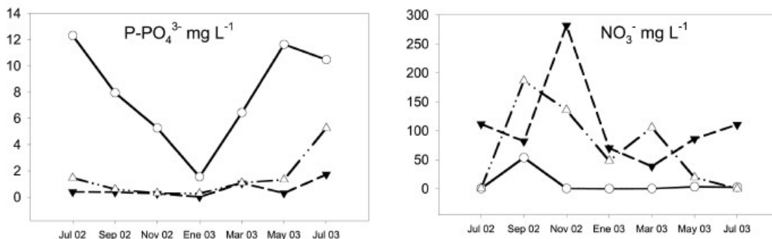
Figura 79: Concentraciones de fosfatos y nitratos en las ramblas de Miranda y El Miedo. Los círculos corresponden a la rambla del Miedo, los triángulos blancos a la rambla del Albuñón y los triángulos negros a la rambla de Miranda (Álvarez-Rogel, Jiménez-Cárceles, FJ, & Nicolás, 2006)
