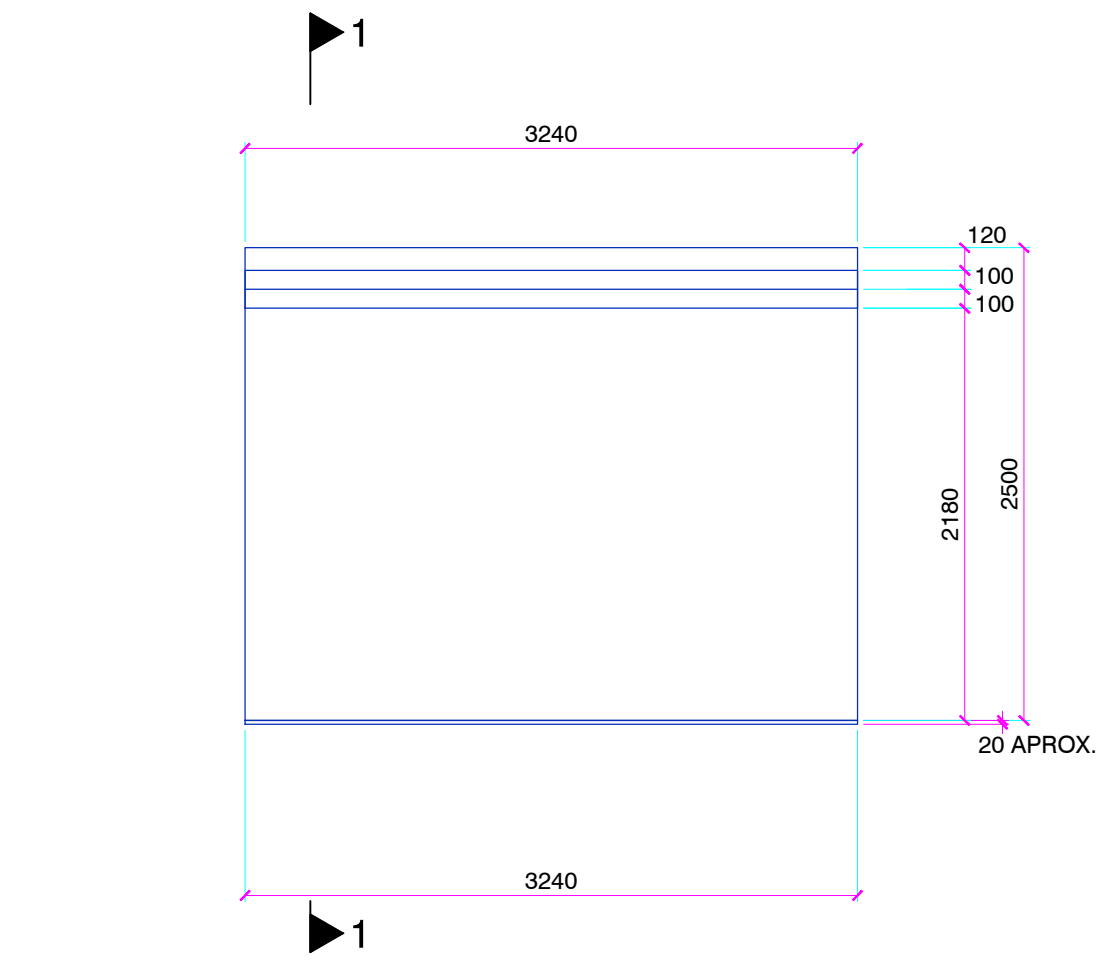
ALZADO DESDE INTERIOR
