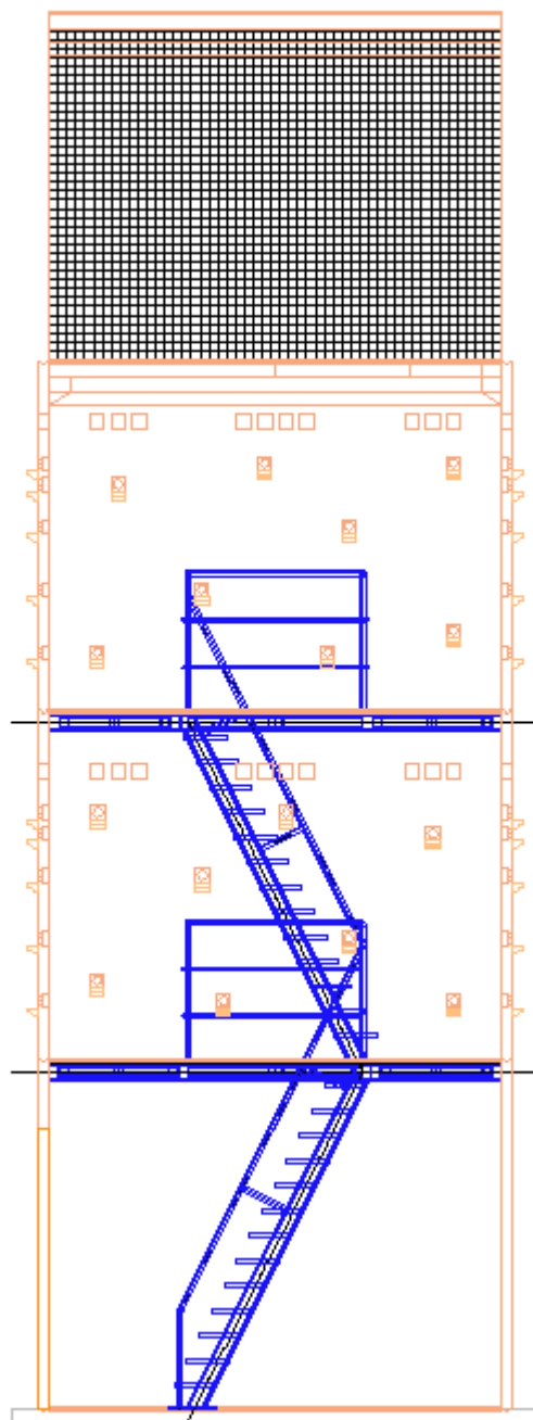
Figura 4: Sección en alzado por escaleras
