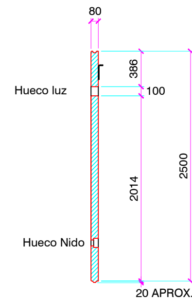
SECCIÓN 1
