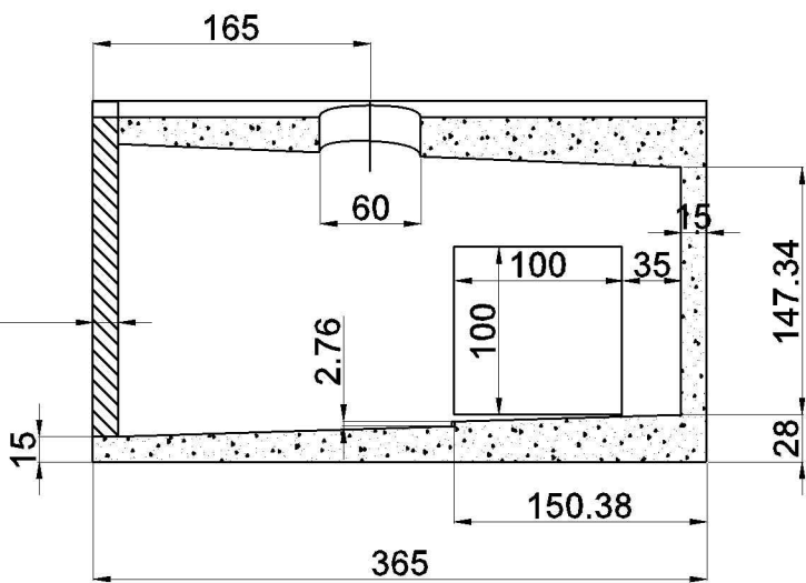
SECCIÓN A-A
