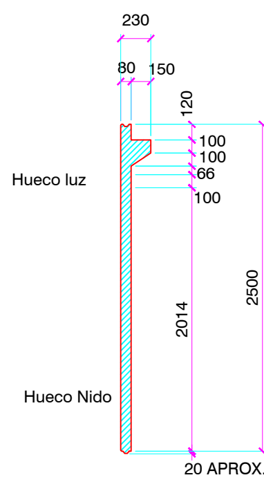
SECCIÓN 1
