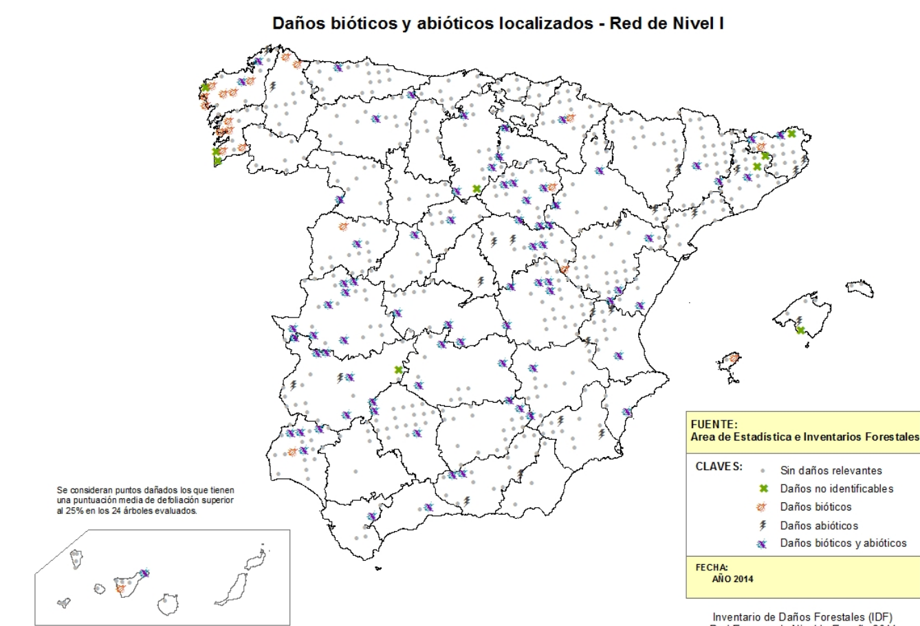
Figura 2 – Puntos con daños (la defoliación media supera el 25%) – IDF España, 2014
