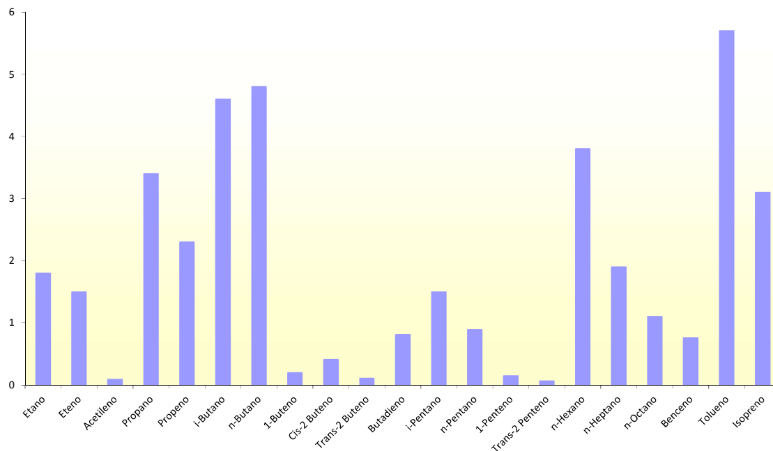
Figura 20. Datos de compuestos orgánicos volátiles en el año 2021
