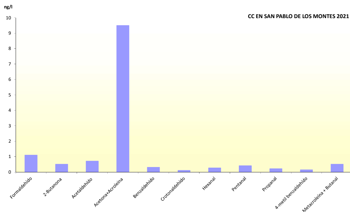
Figura 21. Datos de compuestos carbonílicos en el año 2021
