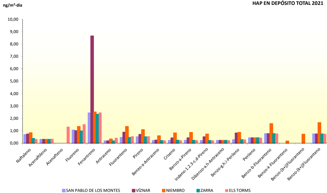
Figura 18. Datos de HAP en depósito total en el año 2021
