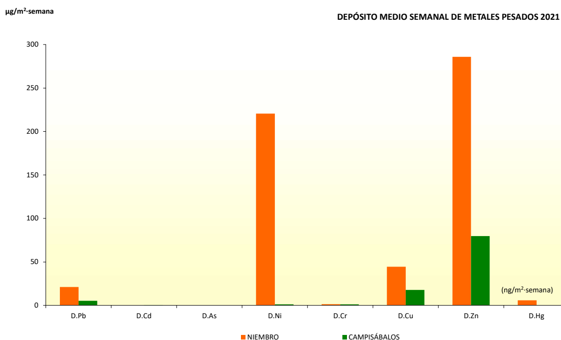
Figura 15. Depósito húmedo semanal de metales pesados durante 2021
