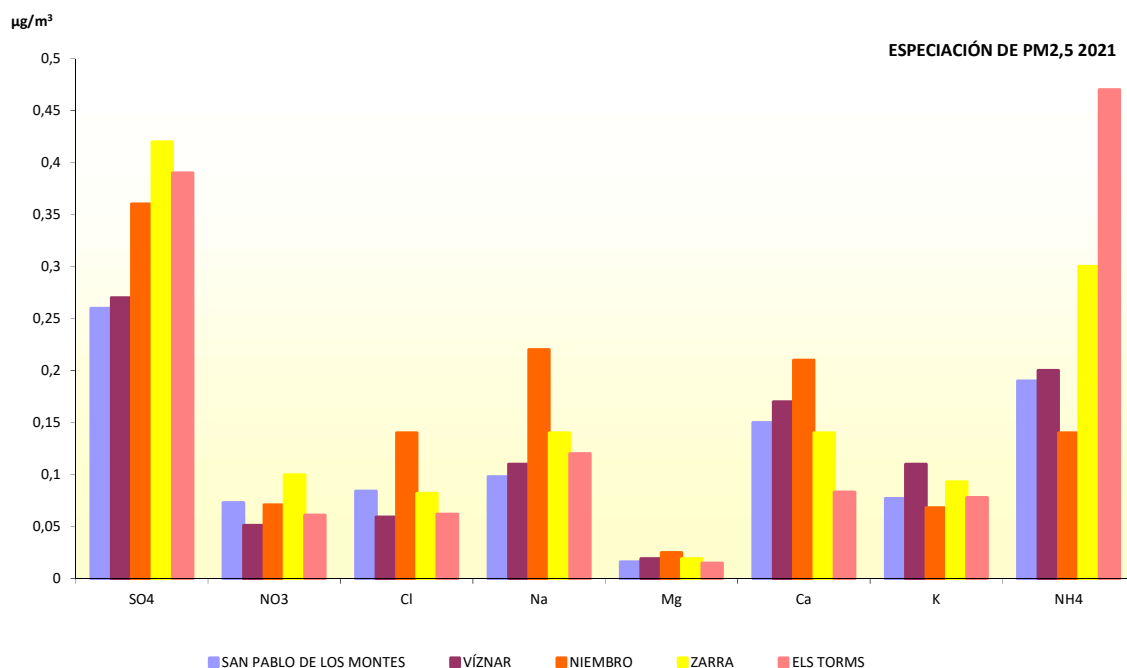
Figura 10. Datos medios anuales de especiación de PM 2,5 en 2021
