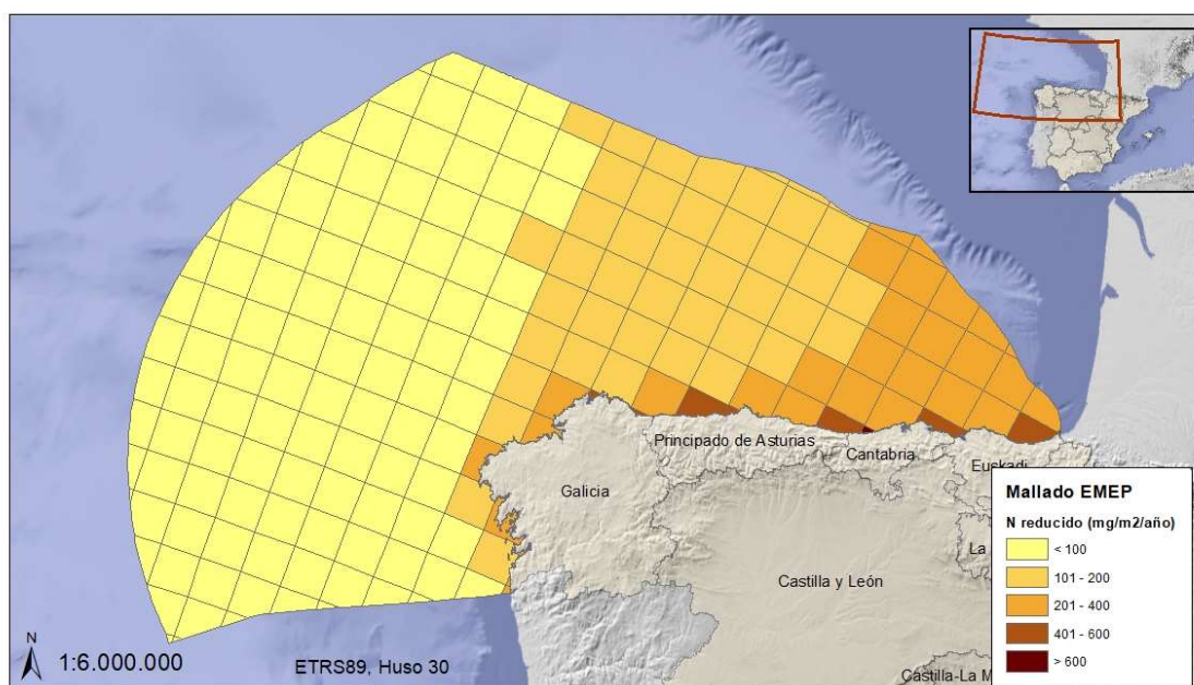
Figura 27. Masa de nitrógeno reducido depositado desde la atmósfera por unidad de superficie durante el año 2014 (Fuente: Figura elaborada por el CEDEX a partir de datos del Programa EMEP)
