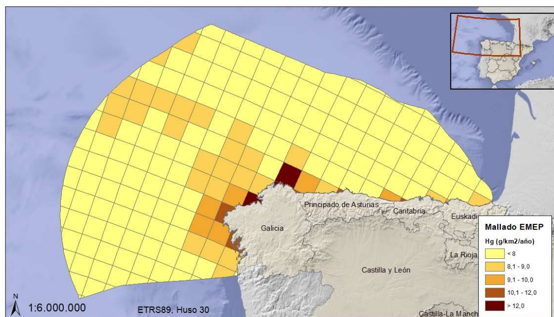
Figura 79. Masa de mercurio depositado desde la atmósfera por unidad de superficie durante el año 2014 (Fuente: Figura elaborada por el CEDEX con datos del Programa EMEP)
