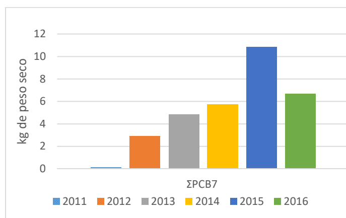
Figura 70. Aportes de PCB's \Sigma 7 congéneres IUPAC (Kg/año) contenidos en los vertidos al mar procedentes de los dragados portuarios (Fuente: Figura elaborada por el CEDEX a partir de datos del Inventario de dragados de Puertos del Estado y de la información aportada por las Capitanías Marítimas y CCAA)
