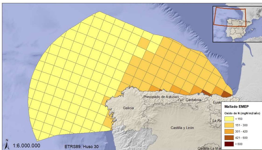
Figura 26. Masa de nitrógeno oxidado depositado desde la atmósfera por unidad de superficie durante el año 2014 (Fuente: Figura elaborada por el CEDEX a partir de datos del Programa EMEP)
