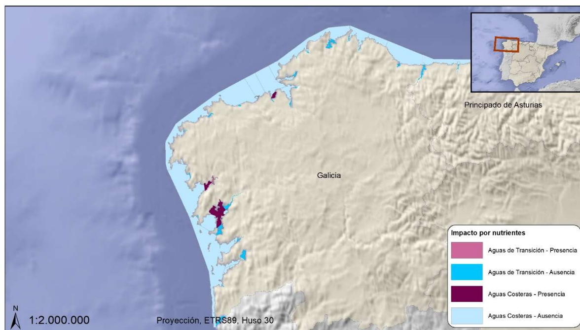
Figura 29. Masas de agua costeras y de transición impactadas por nutrientes – Galicia Costa (Fuente: Mapa elaborado por el CEDEX con datos de la Dirección General del Agua)
