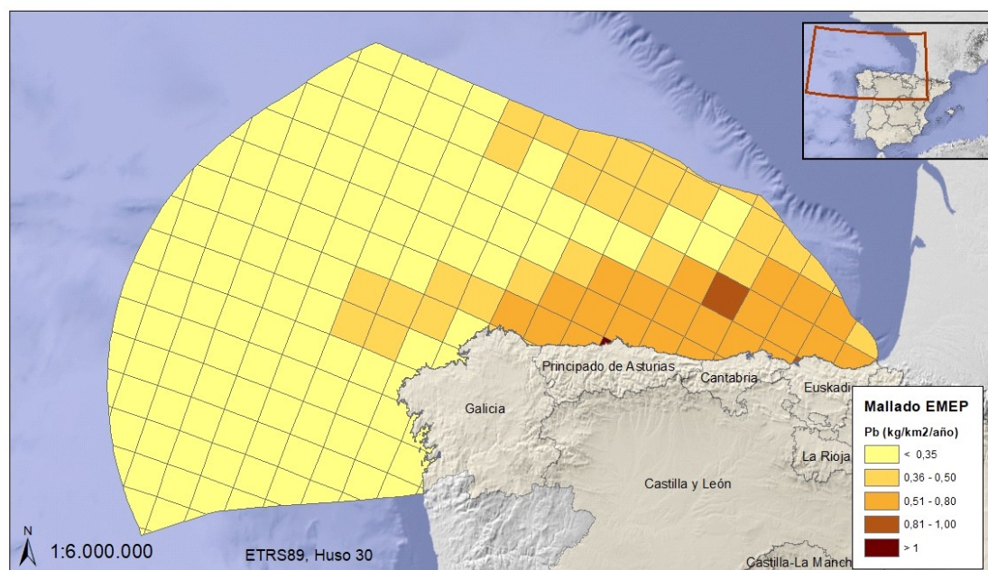
Figura 78. Masa de plomo depositado desde la atmósfera por unidad de superficie durante el año 2014 (Fuente: Figura elaborada por el CEDEX con datos del Programa EMEP)
