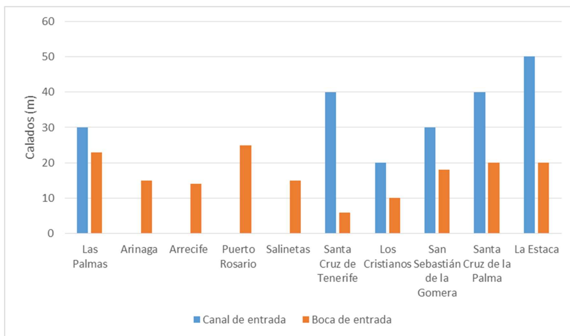
Figura 59. Calados del canal de acceso y de la boca de entrada de los Puertos de Interés General en 2016. (Fuente: Figura elaborada por el CEDEX a partir de datos de Puertos del Estado 26 ).
