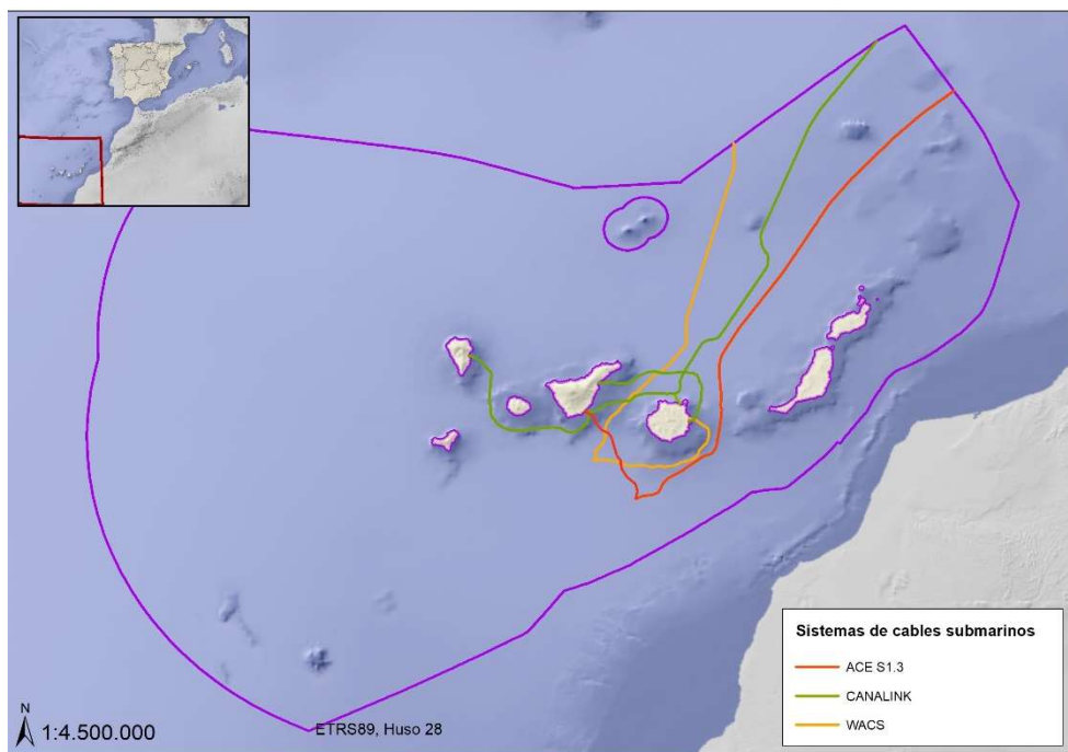
Figura 31. Localización aproximada de los sistemas de cables submarinos puestos en servicio en el periodo 2011-2016. Figura elaborada por el CEDEX a partir de información procedente de la Cartografía Náutica producida por el Instituto Hidrográfico de la Marina (IHM) 12
