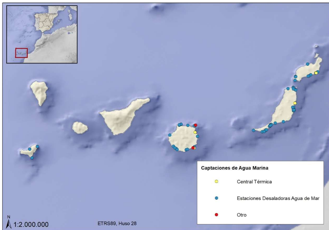
Figura 24. Distribución espacial de las principales captaciones de agua de mar. Fuente: Figura elaborada por el CEDEX a partir del Plan hidrológico de Canarias. Ciclo de Planificación Hidrológica 2015-2021
