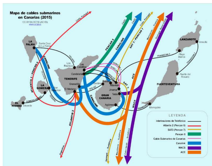
Figura 30. Mapa de cables submarinos de telecomunicaciones en Canarias (2015). Fuente: Observatorio Canario de las Telecomunicaciones y de la Sociedad de la Información 11 .
