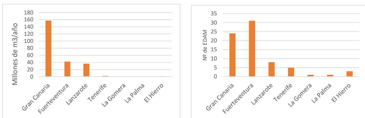
Figura 23. Caudales de agua de mar captados para desalación (izquierda) y número de Estaciones Desaladoras de Agua de Mar (EDAM) contempladas (derecha).
