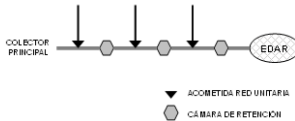
Figura 1 - Cámaras de retención en línea
