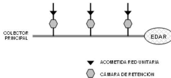
Figura 2 - Cámaras de retención fuera de línea
