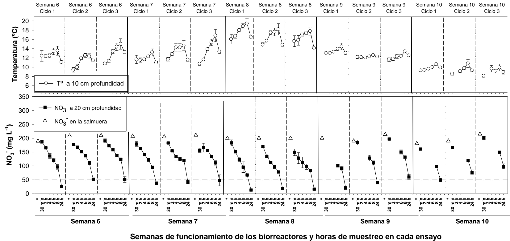
Figura 38. Concentraciones de \text{NO}_3^- en la salmuera (triángulos blancos) y en el interior de los biorreactores rectangulares (cuadrados negros), semanas 6 a 10. También se ha incluido la evolución de la temperatura dentro de los biorreactores. Los valores son la media de los tres biorreactores \pm SD.
