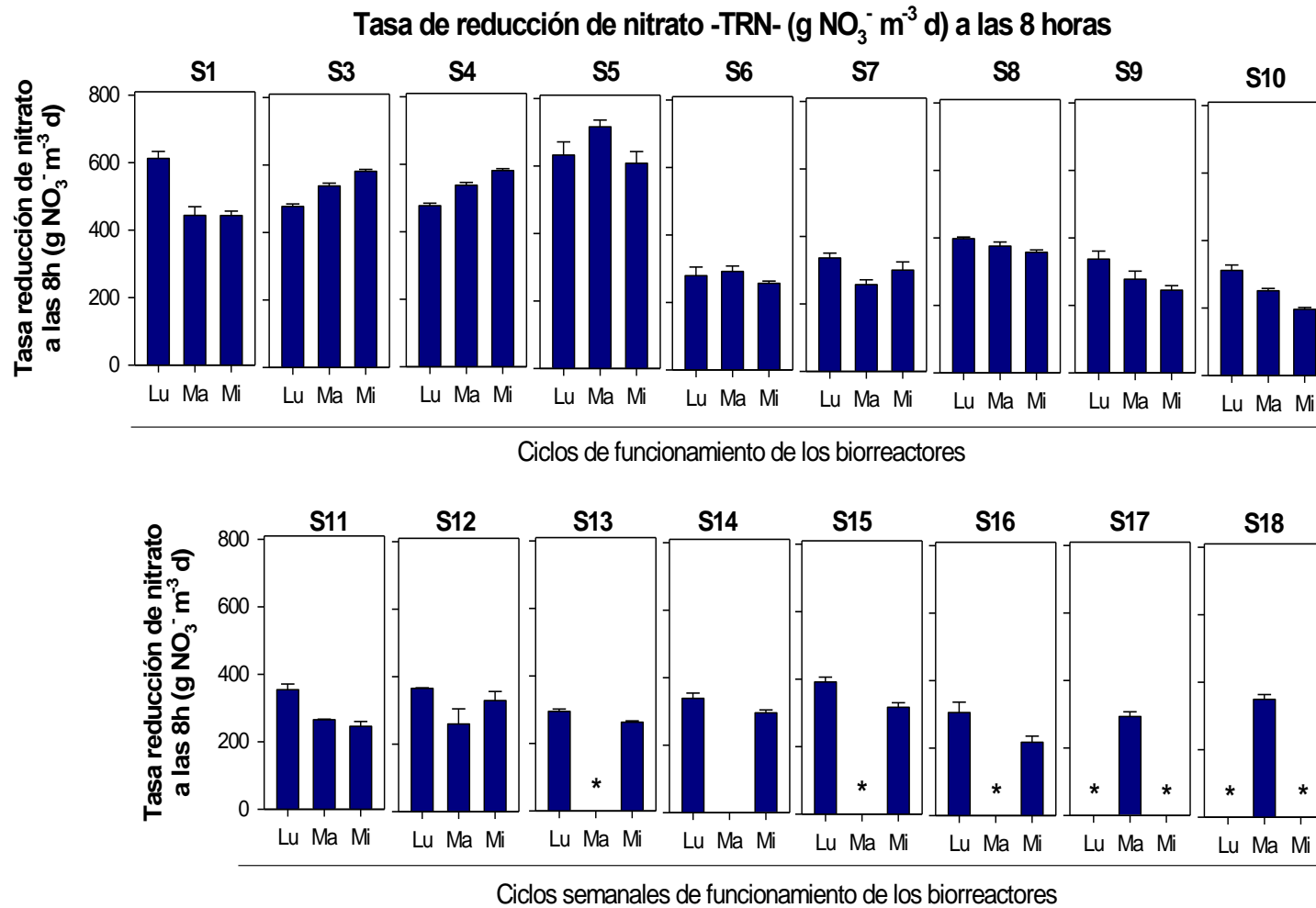
Figura 46. Tasas de reducción de \text{NO}_3^- ( \text{g NO}_3^- \text{m}^{-3} \text{d} ) a las 8 h de TRH en los biorreactores rectangulares. Los valores son la media de los tres biorreactores \pm SD.
