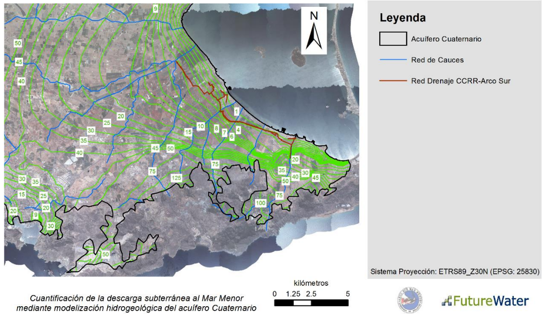
Figura 39. Piezometría calculada para condiciones de año medio (fecha representada 15/03/2004). Zoom a la zona de estudio CRRAS.
