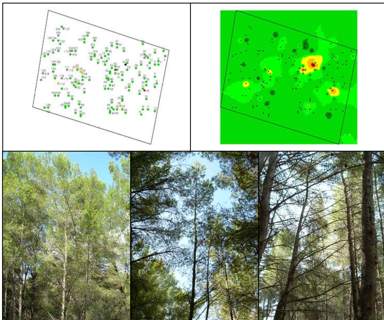
FIG 8: Distribución y modelo de defoliaciones. Defoliación 20%, 30% y 85%
