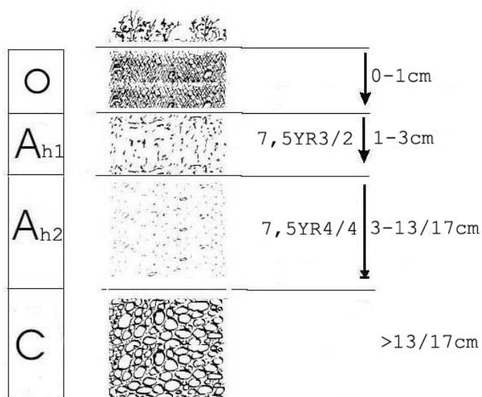
FIG 5: Esquema del perfil 4 del suelo Eutric Leptosol, fase rúbrica de la parcela 41Ph
