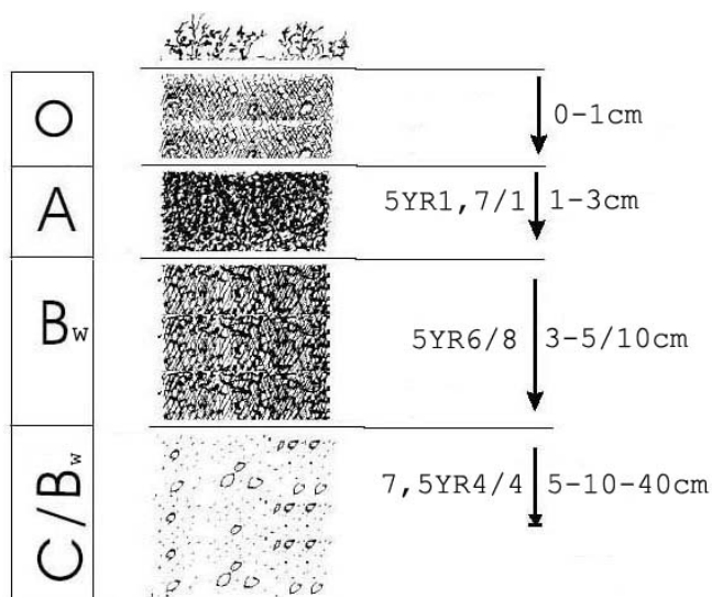
FIG 3: Esquema del perfil 2 del suelo Eutric Leptosol , fase rúdica de la parcela 41Ph
