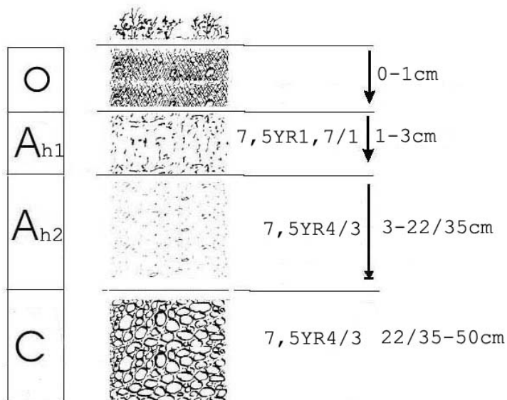
FIG 4: Esquema del perfil 3 del suelo Eutric Leptosol, fase rúdica de la parcela 41Ph
