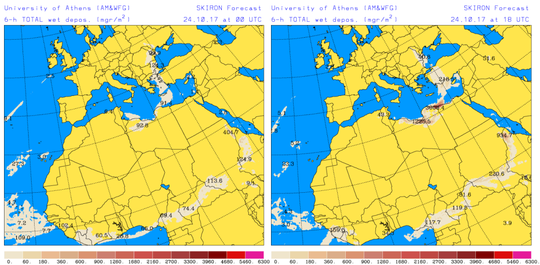
Depósito húmedo de polvo ( \text{mg}/\text{m}^2 ) predicho por el modelo SKIRON para el día 24 de octubre de 2017 a las 00 UTC (izquierda) y a las 18 UTC (derecha). © Universidad de Atenas.
