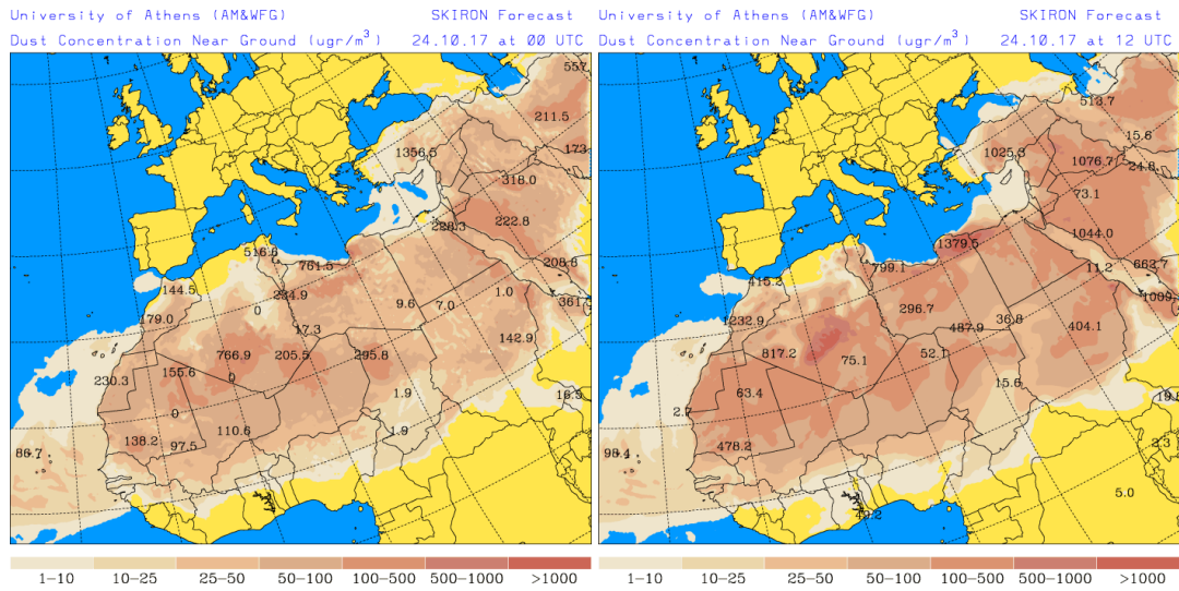
Concentración de polvo ( \mu\text{g}/\text{m}^3 ) predicha por el modelo SKIRON para el día 24 de octubre de 2017 a las 00 UTC (izquierda) y a las 12 UTC (derecha). © Universidad de Atenas.
