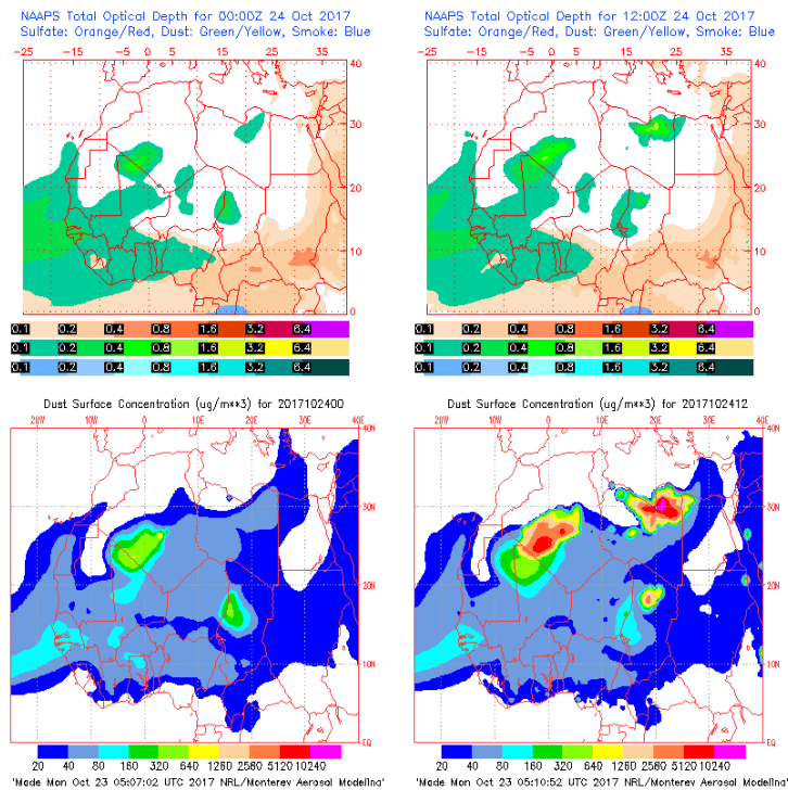
Espesor óptico de aerosoles a 550 nm (arriba) y concentración de polvo a nivel de superficie (abajo) previstos por el modelo NAAPs para el día 24 de octubre de 2017 a las 00 UTC y a las 12 UTC. ©Naval Research Laboratory (NRL), Monterey, CA.
