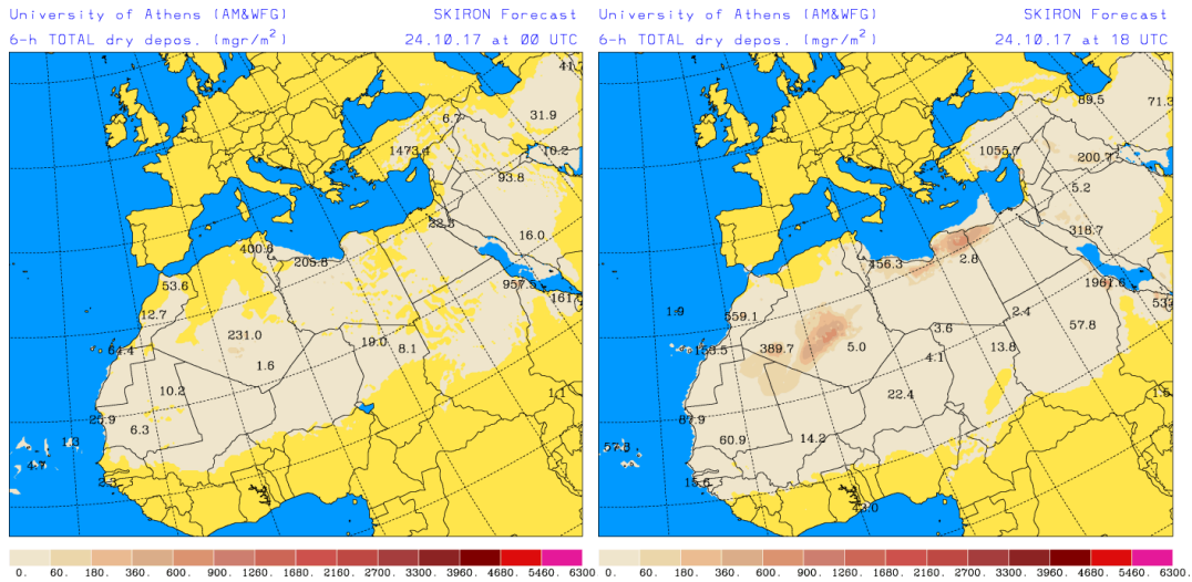
Depósito seco de polvo ( \text{mg}/\text{m}^2 ) predicho por el modelo SKIRON para el día 24 de octubre de 2017 a las 00 UTC (izquierda) y a las 18 UTC (derecha). © Universidad de Atenas.
