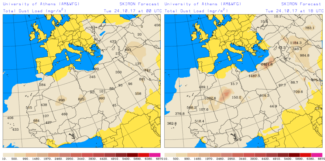
Carga total de polvo ( \text{mg}/\text{m}^2 ) predicha por el modelo SKIRON para el día 24 de octubre de 2017 a las 00 UTC (izquierda) y a las 18 UTC (derecha). © Universidad de Atenas.
