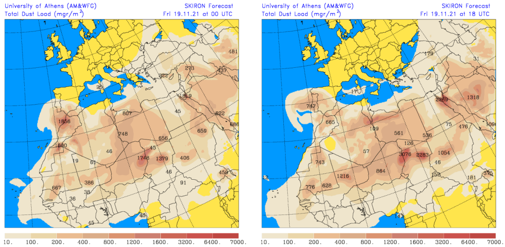
Carga total de polvo ( \text{mg}/\text{m}^2 ) predicha por el modelo SKIRON para el día 19 de noviembre de 2021 a las 00 y 18 UTC © Universidad de Atenas.
