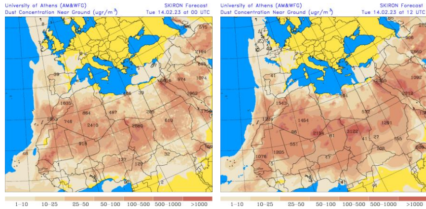
Concentración de polvo ( \mu\text{g}/\text{m}^3 ) predicha por el modelo SKIRON para el día 14 de febrero de 2023 a las 00 y 12 UTC © Universidad de Atenas.
