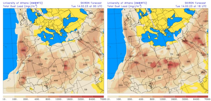
Carga total de polvo ( \text{mg}/\text{m}^2 ) predicha por el modelo SKIRON para el día 14 de febrero de 2023 a las 00 y 18 UTC © Universidad de Atenas.
