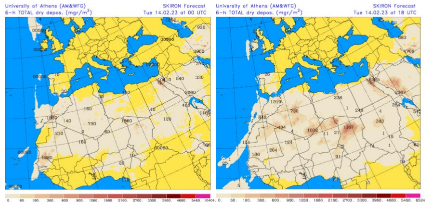
Depósito seco de polvo ( \text{mg}/\text{m}^2 ) predicho por el modelo SKIRON para el día 14 de febrero de 2023 a las 00 y 18 UTC © Universidad de Atenas.
