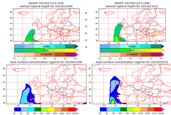
Espesor óptico de aerosoles a 550 nm (arriba) y concentración de polvo a nivel de superficie (abajo) previstos por el modelo NAAPS para el día 14 de febrero de 2023 a las 00 h UTC y a las 12 h UTC. ©Naval Research Laboratory (NRL), Monterey, CA.
