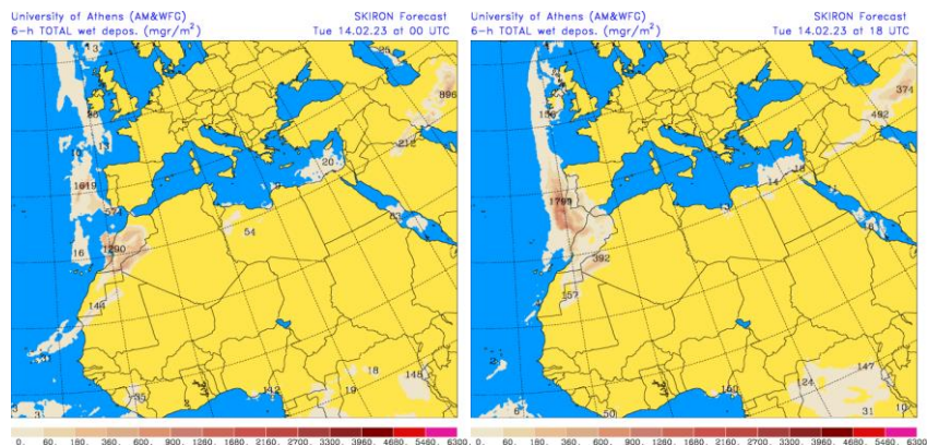
Depósito húmedo de polvo ( \text{mg}/\text{m}^2 ) predicho por el modelo SKIRON para el día 14 de febrero de 2023 a las 00 y 18 UTC © Universidad de Atenas.
