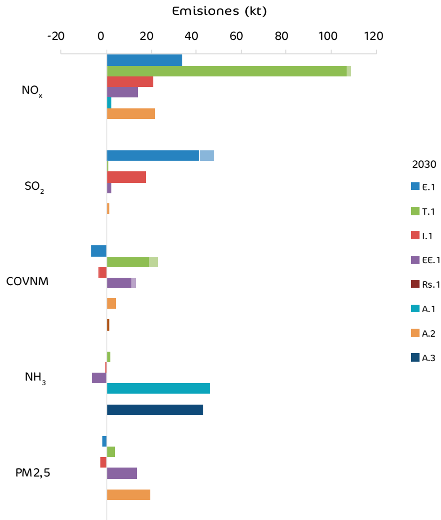
Figura 59. Ahorros y reducciones de emisiones (kt) de los paquetes de medidas del escenario CMA respecto al escenario CM en 2030.
