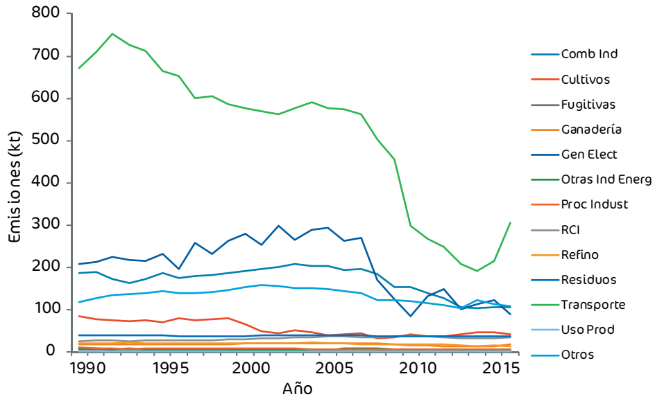
Figura 11. Emisiones de NOx inventariadas con los ajustes aprobados para España (serie 1990-2016), desagregadas por sectores de actividad.
