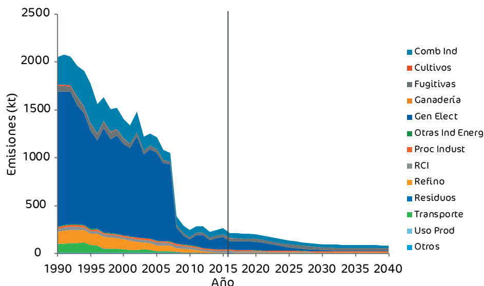
Figura 62. Emisiones de SO 2 inventariadas (serie 1990-2016) y proyectadas (serie 2016-2040) bajo el escenario con medidas adicionales (CMA) desagregado para los principales sectores de actividad.
