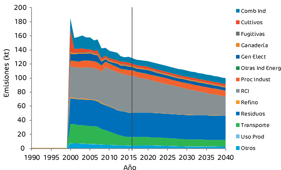
Figura 45. Emisiones de PM 2,5 inventariadas (serie 1990-2016) y proyectadas (serie 2016-2040) bajo el escenario con medidas (CM) desagregado para los principales sectores de actividad.
