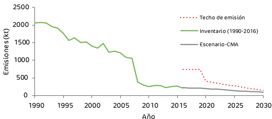
Figura 63. Evolución temporal de las emisiones de SO 2 desde 1990 hasta 2030 y techos de emisión a partir de 2016.
