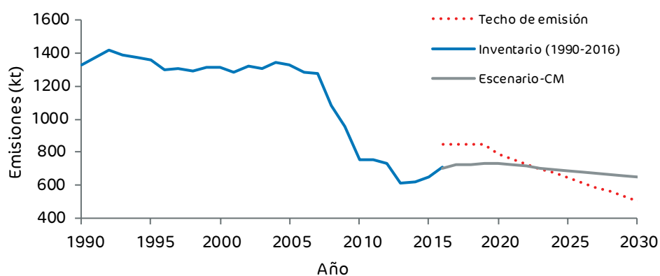
Figura 40. Evolución temporal de las emisiones de NO x desde 1990 a 2016 descontando las emisiones recogidas en el artículo 4.3.d) de la Directiva (UE) 2016/2284y con los ajustes aprobados, proyecciones hasta 2030 y relación con los techos de emisión a partir de 2016.
