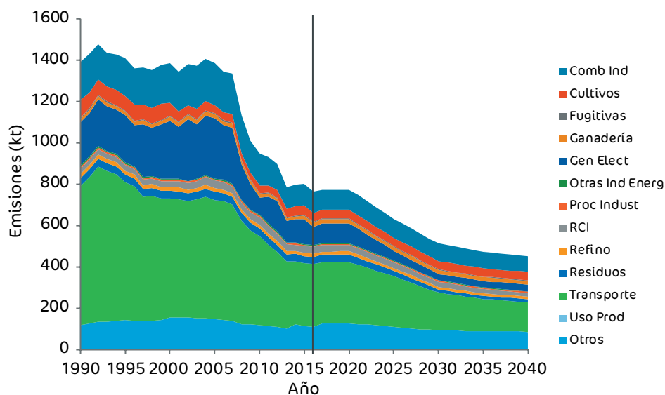
Figura 64. Emisiones de NO x inventariadas (serie 1990-2016) y proyectadas (serie 2016-2040) bajo el escenario con medidas adicionales (CMA) desagregado para los principales sectores de actividad.
