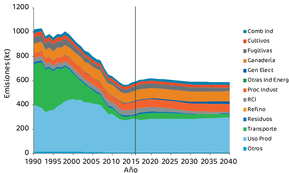
Figura 66. Emisiones de COVNM inventariadas (serie 1990-2016) y proyectadas (serie 2016-2040) bajo el escenario con medidas adicionales (CMA) desagregado para los principales sectores de actividad.
