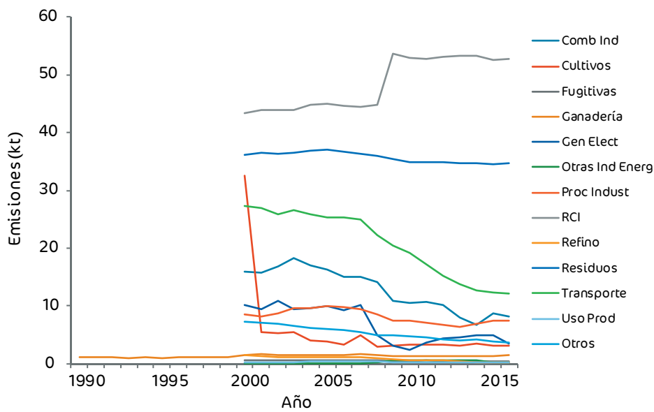
Figura 14. Emisiones de PM 2,5 inventariadas (serie 2000-2016), desagregadas por sectores de actividad.
