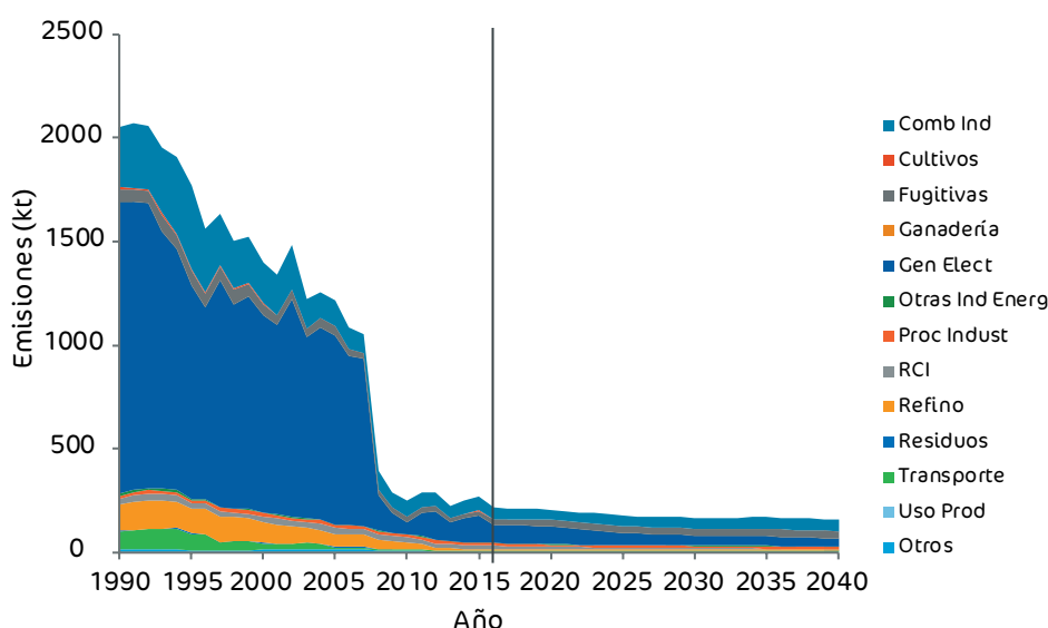
Figura 37. Emisiones de SO 2 inventariadas (serie 1990-2016) y proyectadas (serie 2016-2040) bajo el escenario con medidas existentes (CM) desagregado para los principales sectores de actividad.
