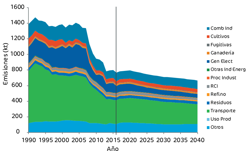
Figura 39. Emisiones de NO x inventariadas (serie 1990-2016) y proyectadas (serie 2016-2040) bajo el escenario con medidas existentes (CM) desagregado para los principales sectores de actividad.
