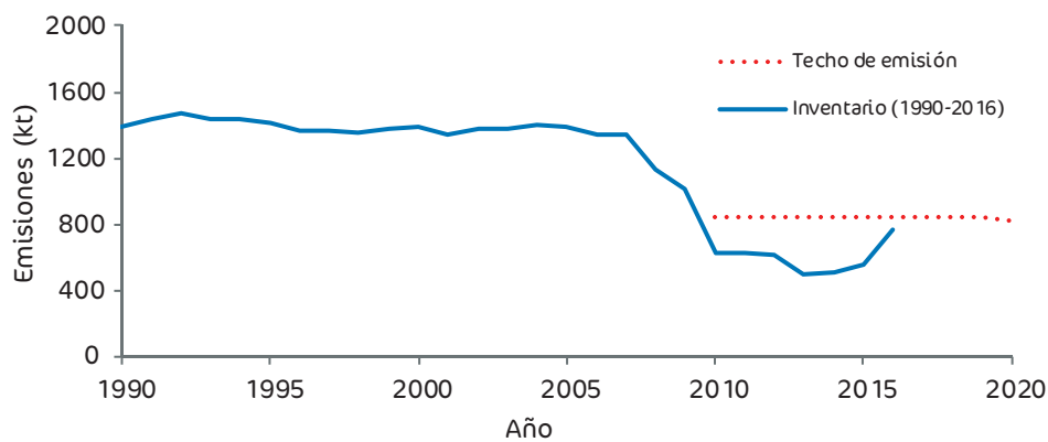
Figura 5. Evolución de las emisiones nacionales inventariadas, sin Islas Canarias, descontando las emisiones recogidas en el artículo 4.3.d) de la Directiva (UE) 2016/2284 y con los ajustes aprobados para NO x (serie 1990-2016), y techos nacionales de emisión comprometidos a partir del año 2010.
