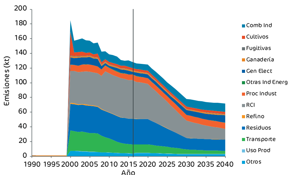
Figura 70. Emisiones de PM 2,5 inventariadas (serie 2000-2016) y proyectadas (serie 2016-2040) bajo el escenario con medidas adicionales (CMA) desagregado para los principales sectores de actividad.
