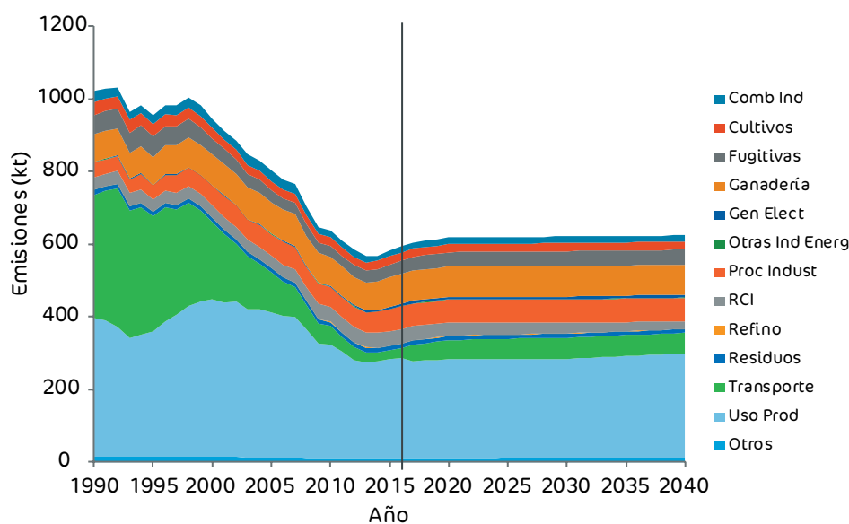
Figura 41. Emisiones de COVNM inventariadas (serie 1990-2016) y proyectadas (serie 2016-2040) bajo el escenario con medidas existentes (CM) desagregado para los principales sectores de actividad.
