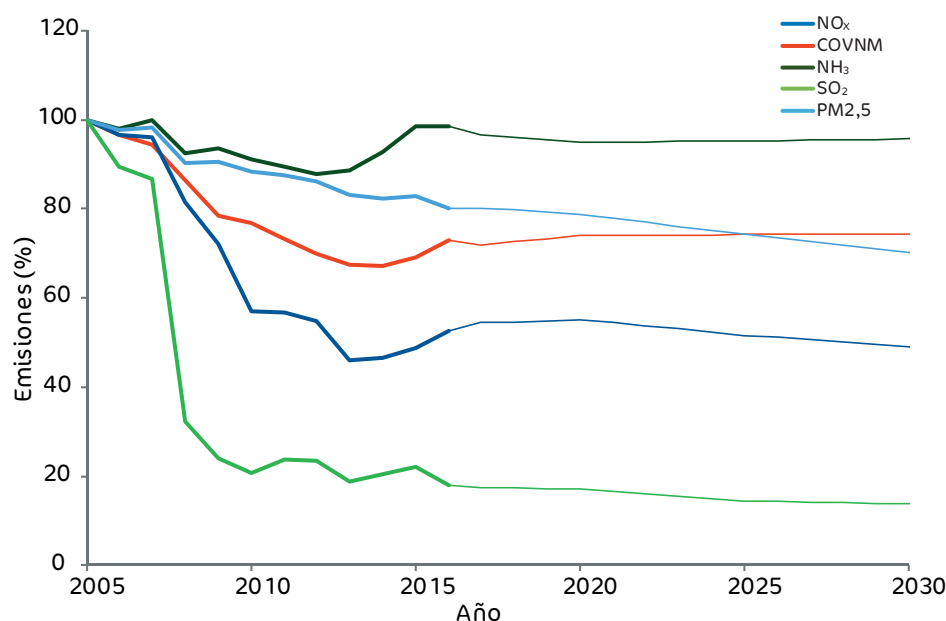
Figura 36. Evolución temporal de las emisiones de NH 3 , COVNM, NO x , PM2,5 y SO 2 inventariadas y proyectadas para el escenario CM, excluyendo las Islas Canarias, descontando las emisiones recogidas en el artículo 4.3.d) de D 2106/2284 y con los ajustes aprobados para NO x .
