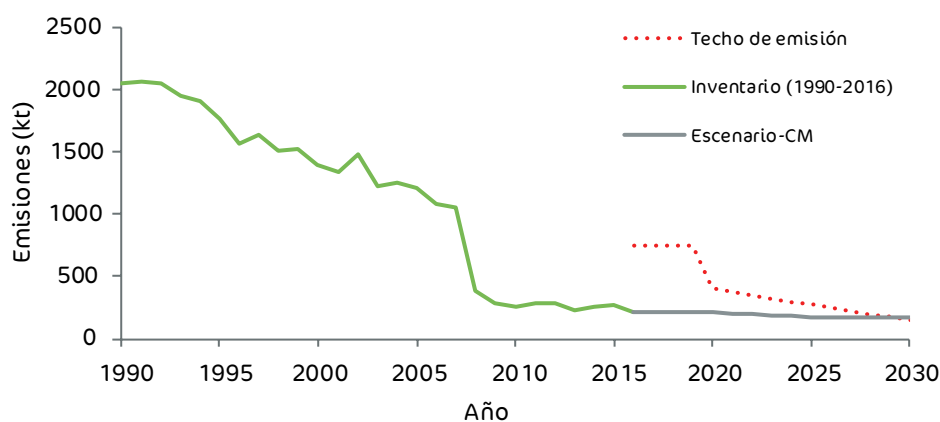
Figura 38. Evolución temporal de las emisiones de SO 2 desde 1990 a 2016 proyecciones hasta 2030 y relación con los techos de emisión a partir de 2016.
