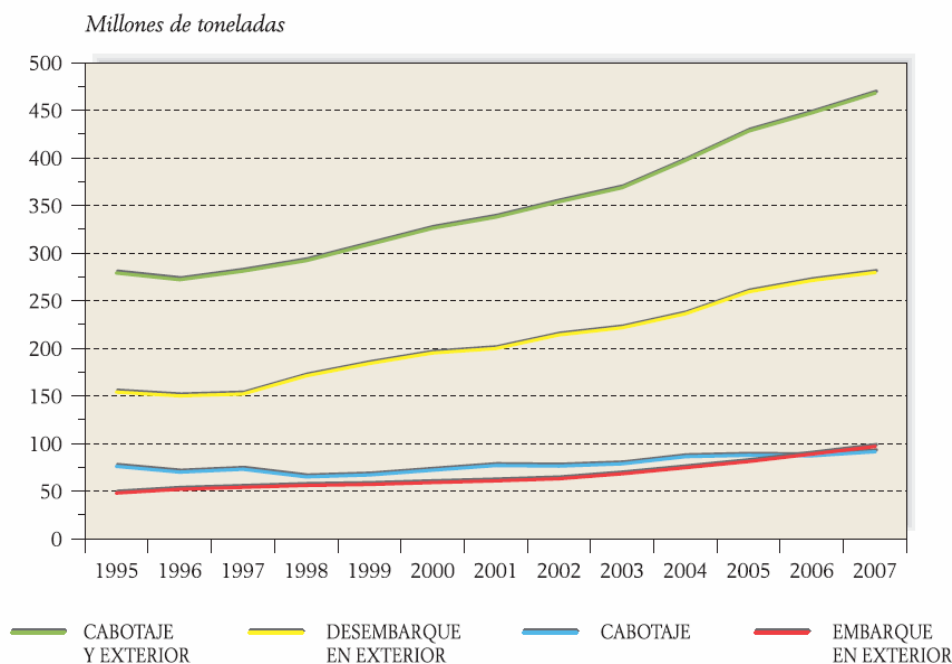
Figura 31: Embarques más Desembarques en cabotaje y exterior
