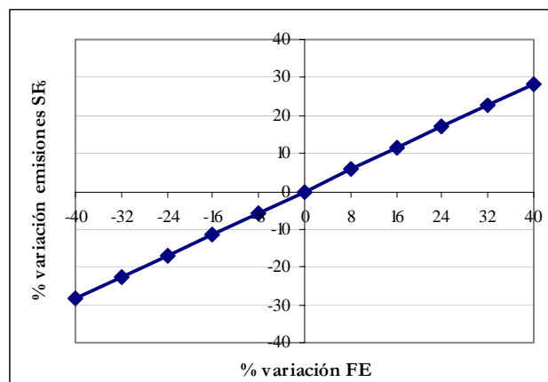
Figura 69. Variación de las emisiones con la variación del factor de emisión en equipos eléctricos.
