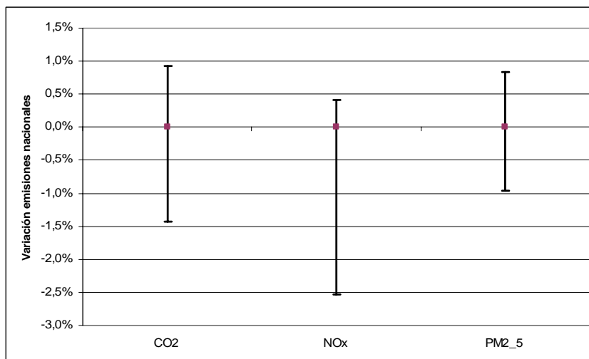
Figura 61. Rango de variación de las emisiones nacionales en relación a la variación más probable de los parámetros del sector transporte por carretera.
