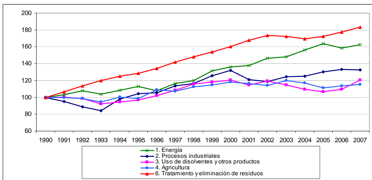
Figura 43: Evolución de las emisiones por grupo de actividad
