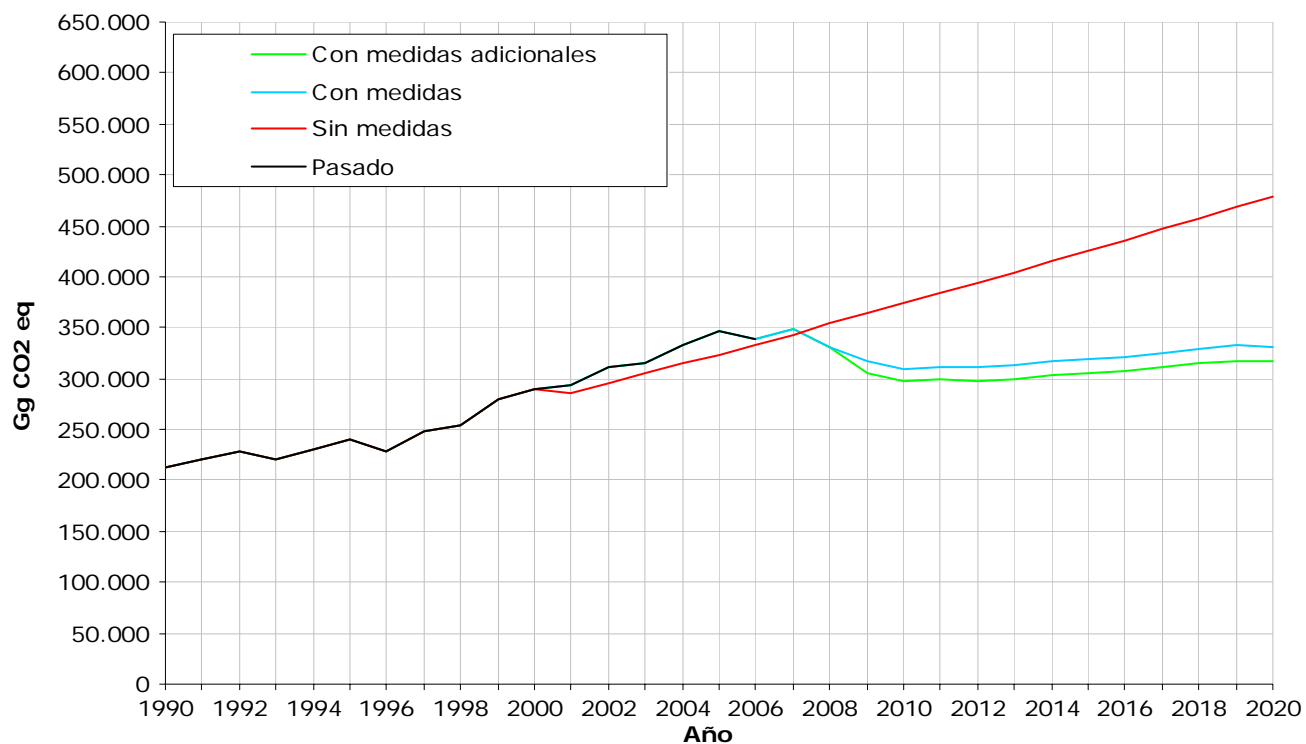
Figura 53. Evolución de las emisiones de CO 2 equivalente para el grupo CRF-1: "Energía".
