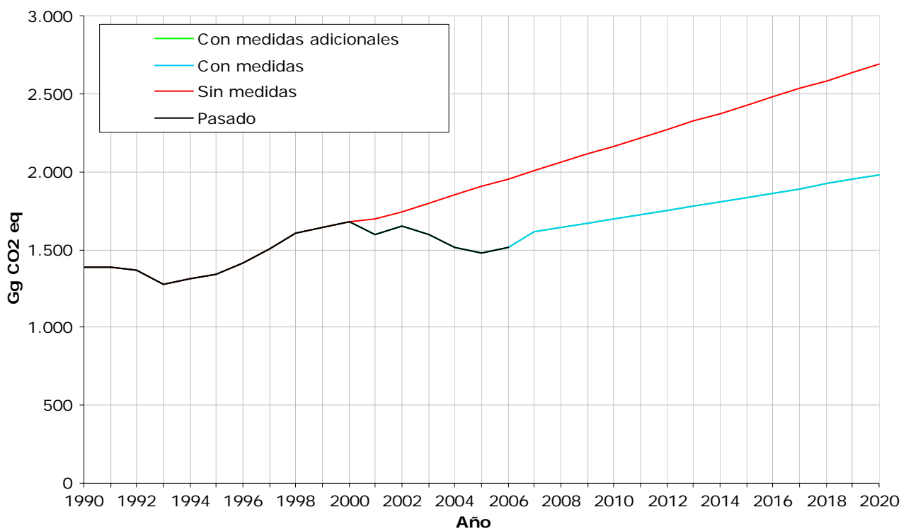
Figura 71. Evolución de las emisiones de CO 2 equivalente para el grupo CRF-3: "Uso de Disolventes".
