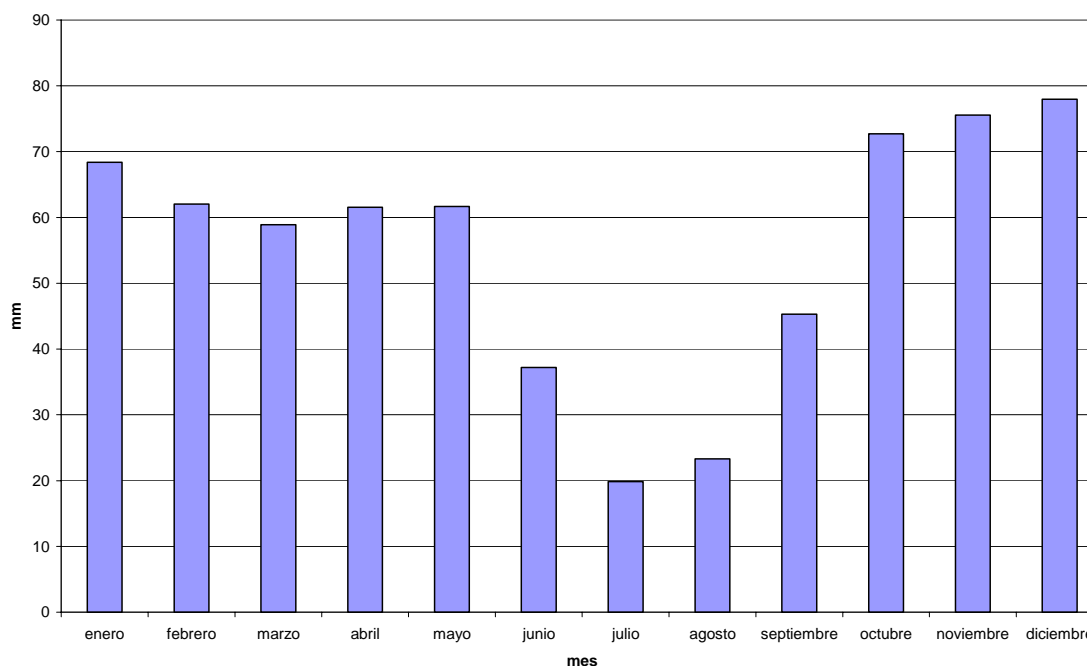
Figura 14: Distribución anual de las precipitaciones medias
