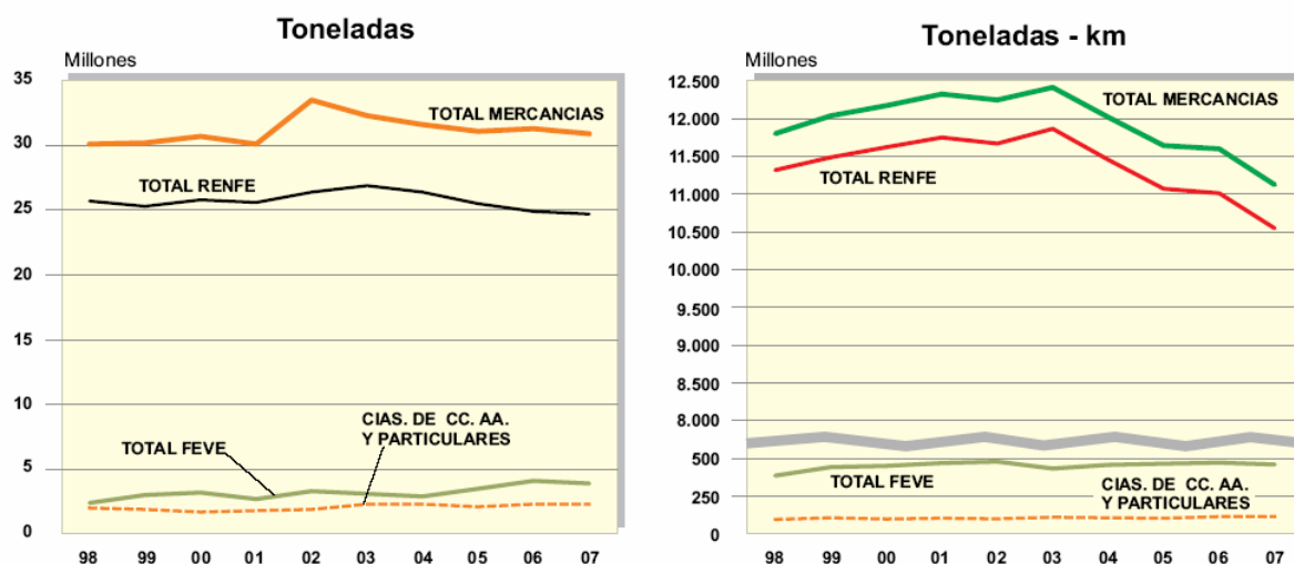
Figura 29: Evolución del transporte ferroviario de mercancías (1998-2007)
