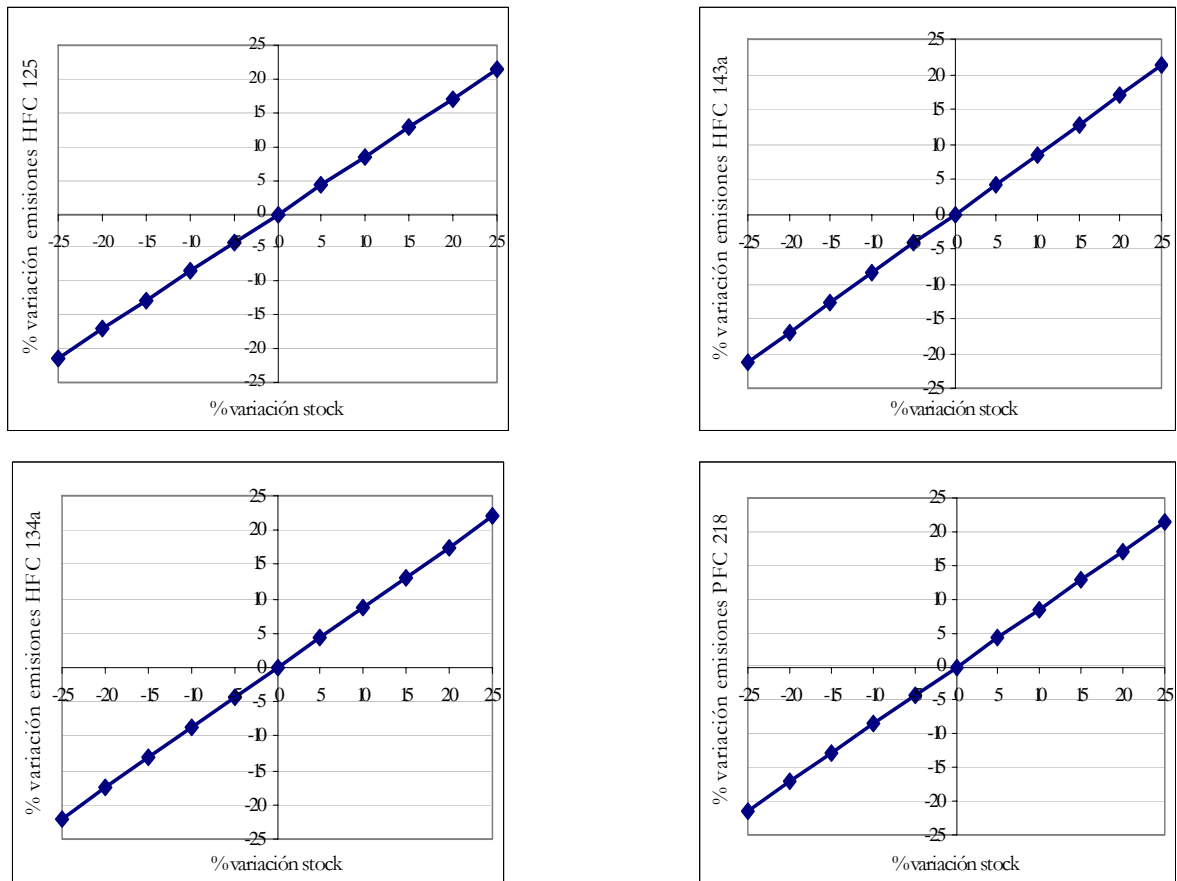
Figura 67. Variación de las emisiones con la variación del stock de HFCs y PFCs, en el sector de equipos de refrigeración.
