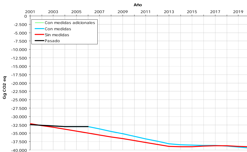
Figura 86: Proyecciones de absorción de CO 2 por los sumideros tras la introducción del PFE.
