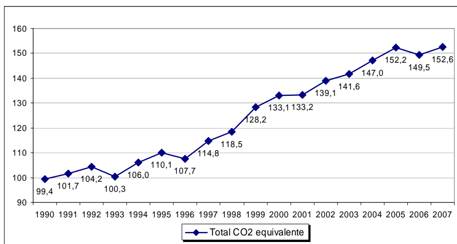
Figura 38: Inventario de gases de efecto invernadero de España. Evolución de las Emisiones. Síntesis de resultados de la edición 1990-2007
