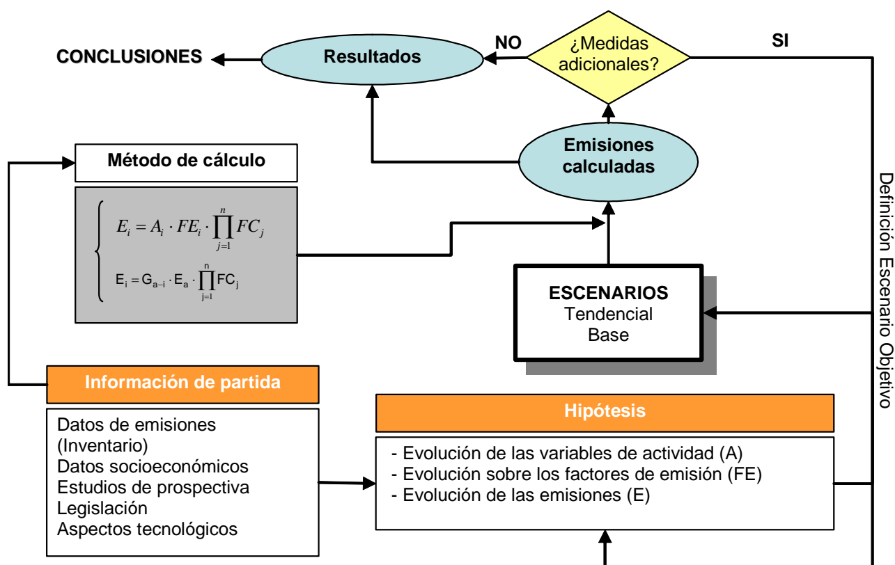
Figura 87. Metodología SEP para el cálculo de proyecciones a nivel de actividad 21 .
