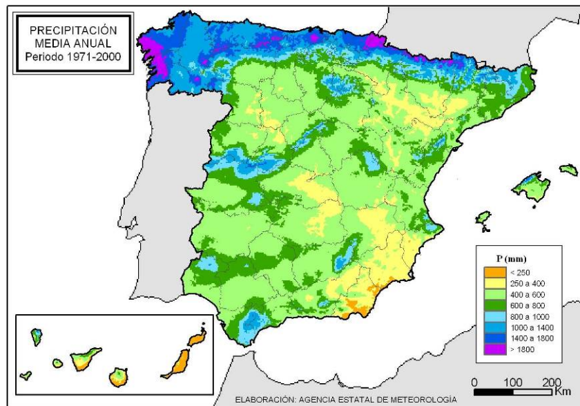
Figura 12: Precipitación media anual (mm) (1971-2000)
