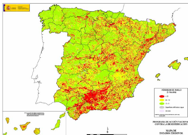
Figura 8: Mapa de Pérdidas de suelo
