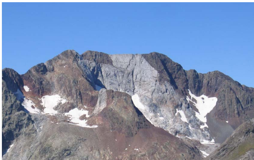
Figura 99: Glaciar septentrional y heleros de los Picos del Infierno. Año 2007
