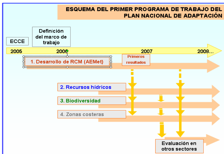
Figura 93: Esquema del Primer Programa de Trabajo del Plan Nacional de Adaptación.
