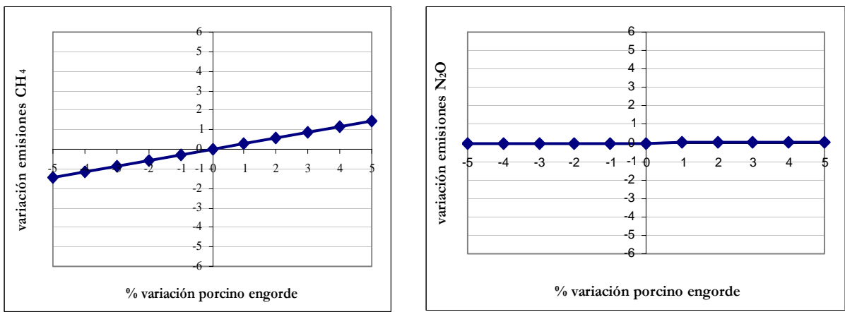
Figura 77. Variación de las emisiones con la variación del número de cabezas de porcino de engorde.
