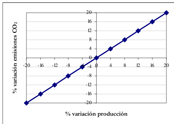
Figura 65. Variación de las emisiones con la variación de la producción total de clínker.
