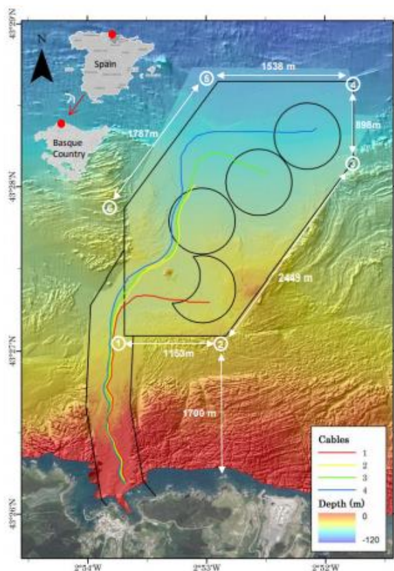
Figura 21. Localización de los sistemas de cables submarinos en BIMEP (Fuente: Bald et al. (2015)) y longitud de los mismos (Fuente: BIMEP)
