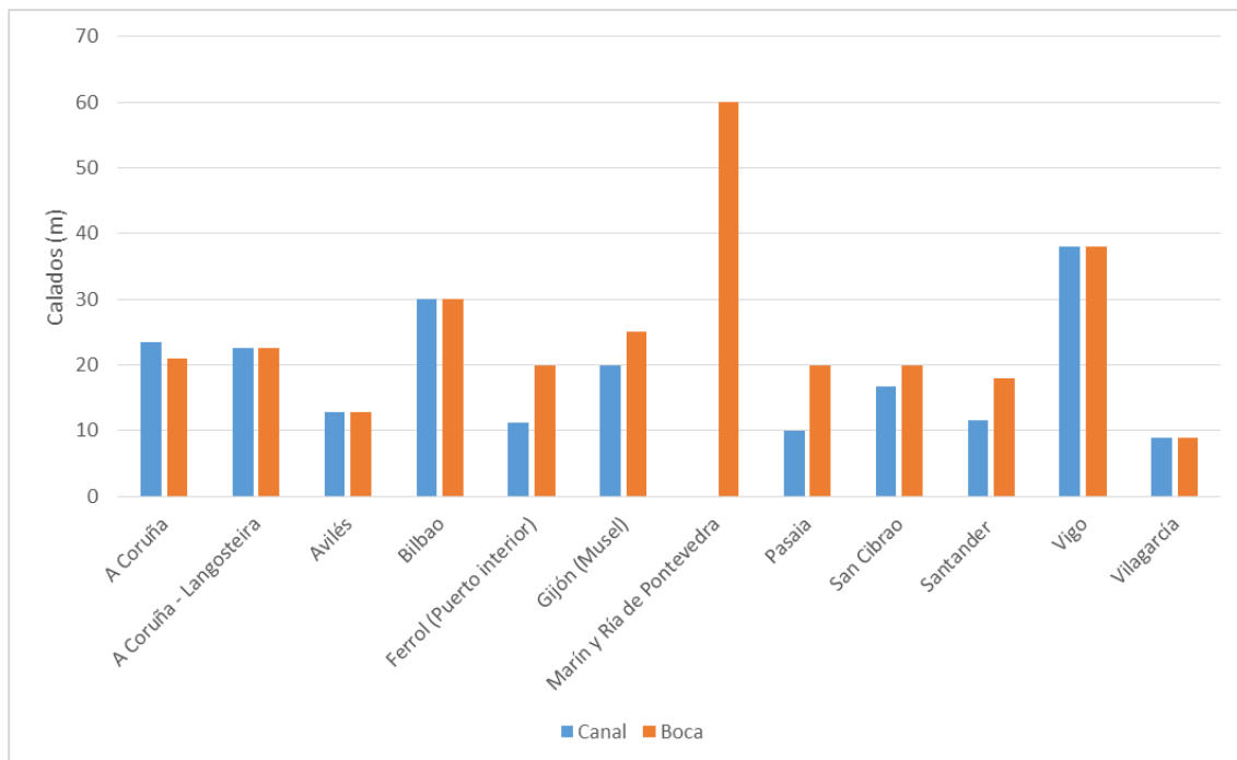
Figura 49. Calados del canal de acceso y de la boca de los Puertos de Interés General en 2016
