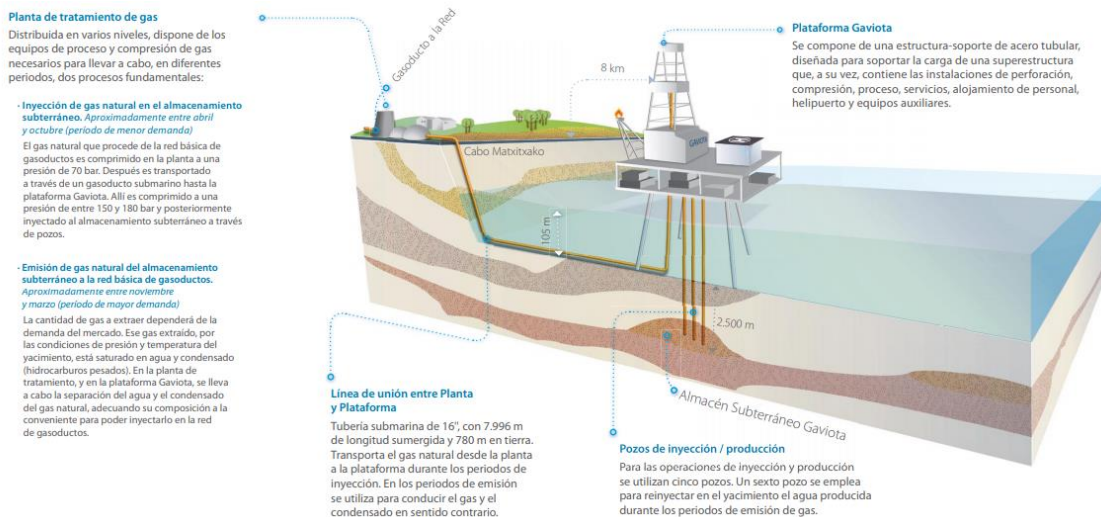
Figura 15. Almacenamiento de gas Gaviota. Fuente: Enagás 2 .
