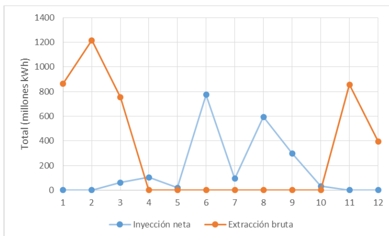
Figura 14. Inyección y extracción del almacenamiento Gaviota para los distintos meses del año 2016. Fuente: Elaborado por el CEDEX a partir de datos de Enagás 1 .
