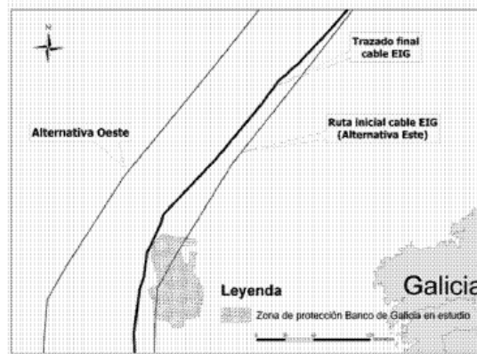
Figura 22. Alternativas y trazado final propuesto para el cable submarino “Europe-India Gateway”.
