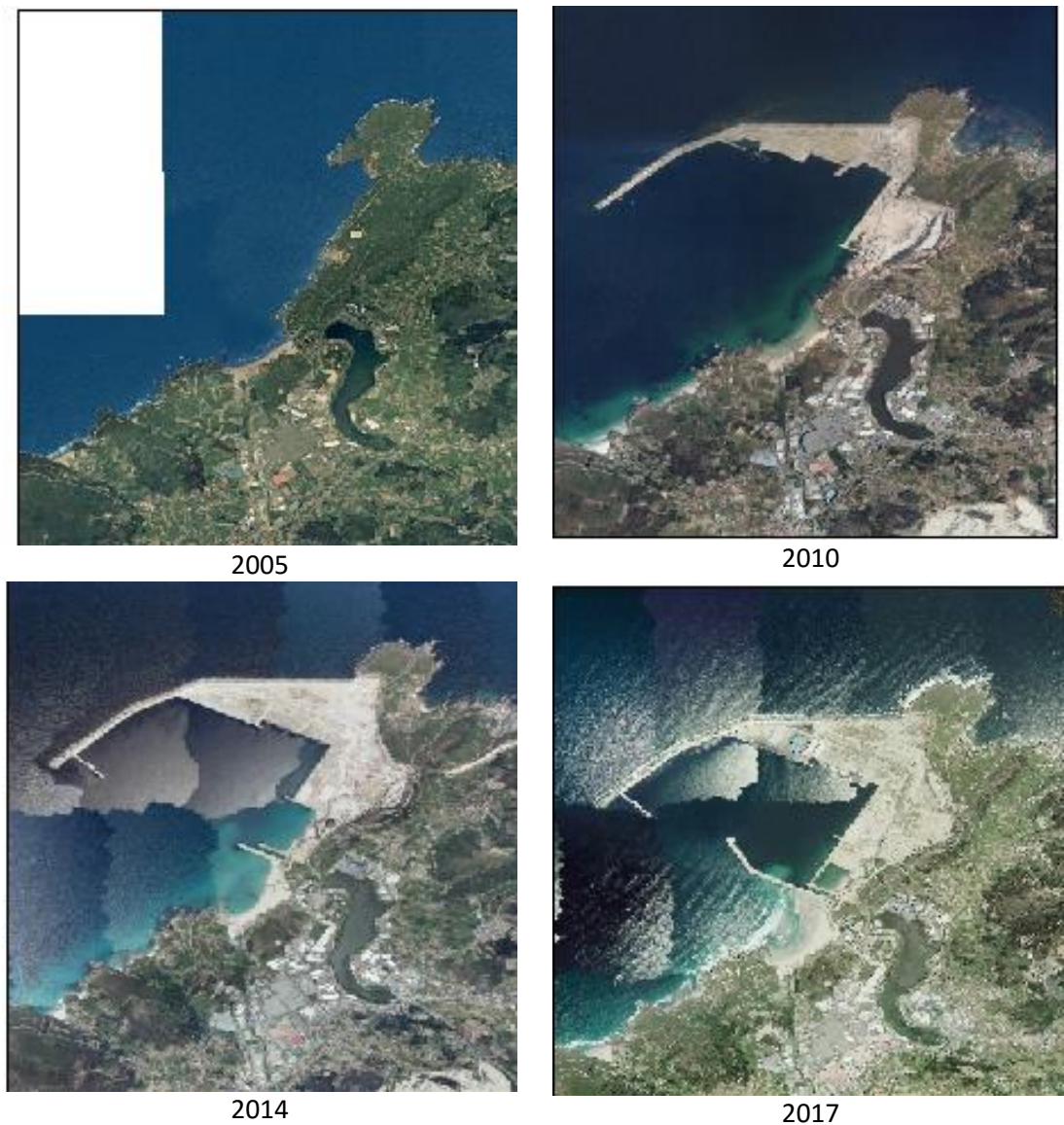
Figura 42. Construcción del puerto de Langosteira. Fuente: Plan Nacional de Ortofotografía Aérea
