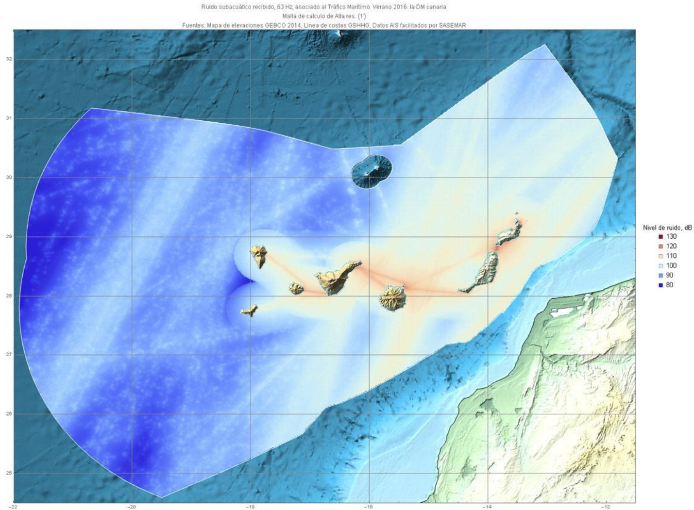
Figura 20 Niveles medio de ruido recibido dB re 1 \mu Pa en verano de 2016, 63 Hz
