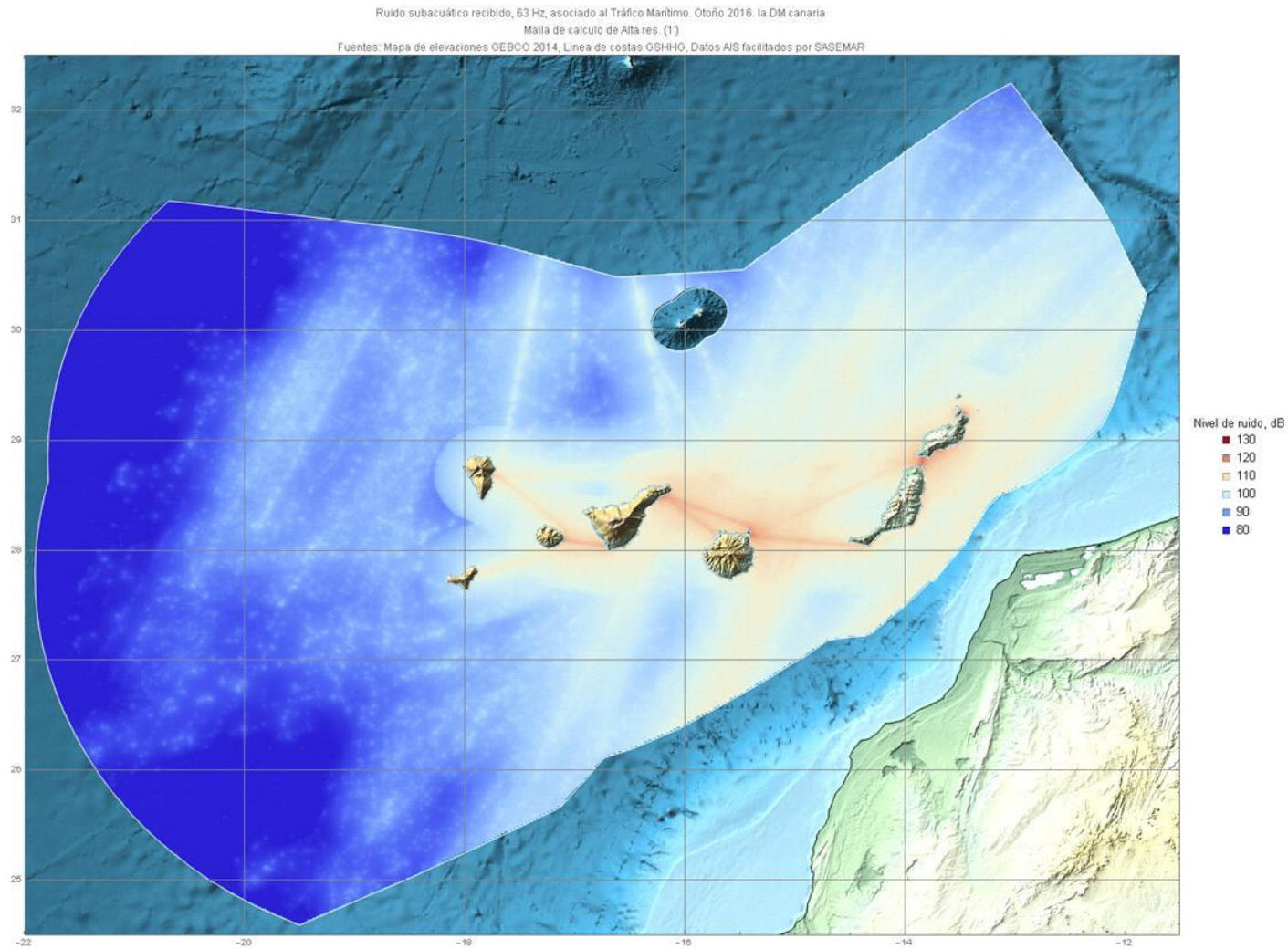
Figura 21. Niveles medio de ruido recibido dB re 1 \mu Pa en otoño de 2016, 63 Hz
