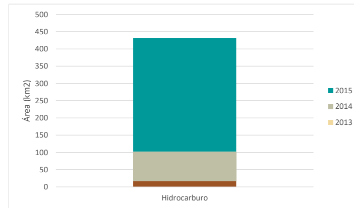
Figura 8. Área de los incidentes de contaminación seleccionados para el periodo 2013-2016
