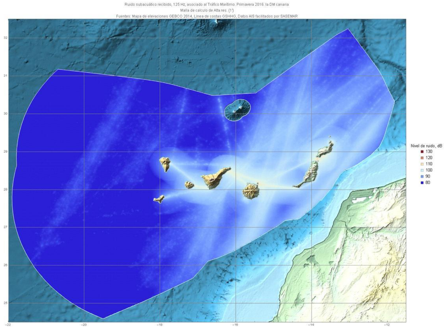
Figura 23. Niveles medio de ruido recibido dB re 1 \mu Pa en primavera de 2016, 125 Hz
