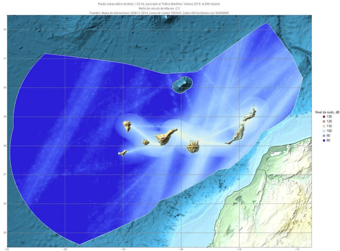
Figura 24. Niveles medio de ruido recibido dB re 1 \mu Pa en verano de 2016, 125 Hz
