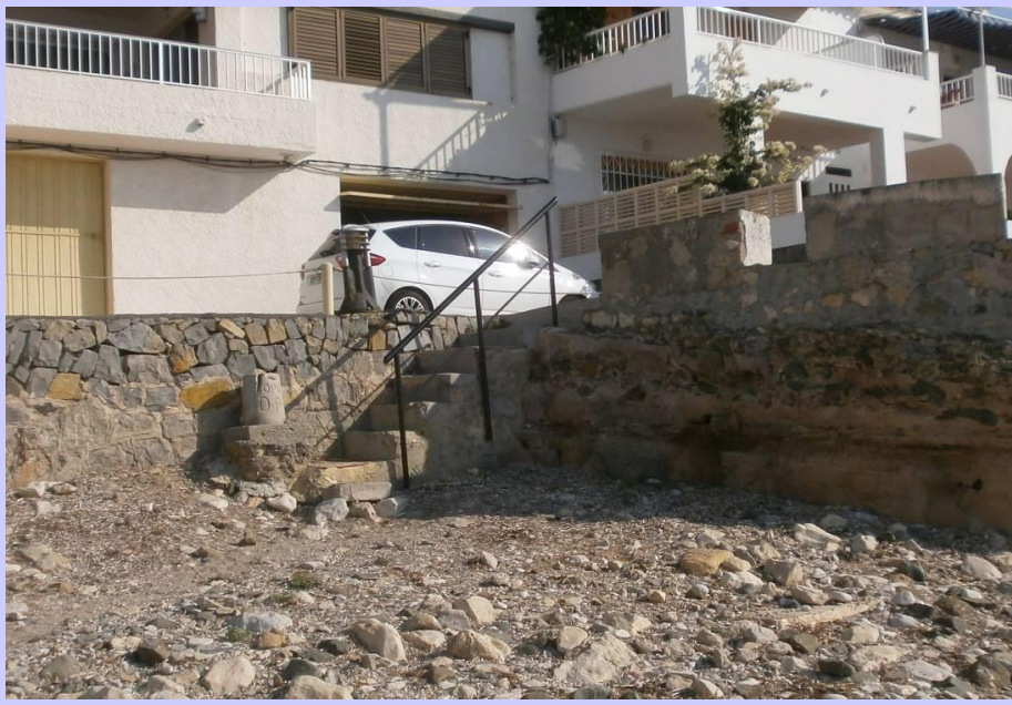
Imágenes del antes y el después de una de las escaleras
