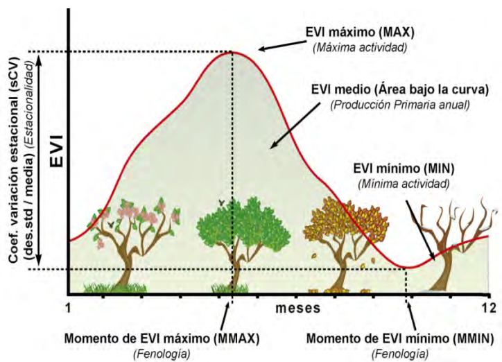
Fig. 08: Curva anual de la dinámica del índice de verdor (EVI o NDVI) e indicadores del funcionamiento derivados de su parametrización.
