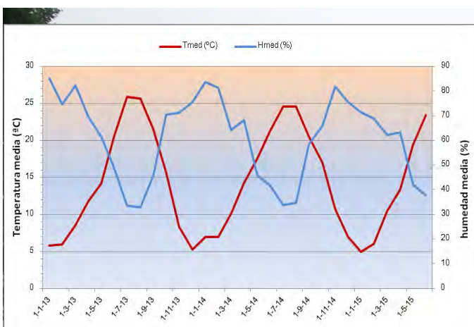
Fig. 04: Comportamiento cíclico de temperatura y humedad media para la serie histórica disponible en el P.N. de Cabañeros.
