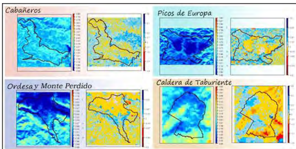
Fig. 09: Ejemplos de mapa de índice de verdor medio en el periodo 2001/2014 (izquierda) y las anomalías respecto a este (derecha) en distintos parques de cada región biogeográfica, correspondientes a diciembre de 2014 (compuesto 22).
