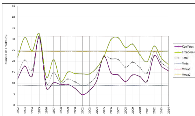
Fig. 05: Evolución interanual de la defoliación en porcentaje de árboles dañados, tanto para coníferas (en violeta) como frondosas (en verde), durante el periodo 1992-2014
